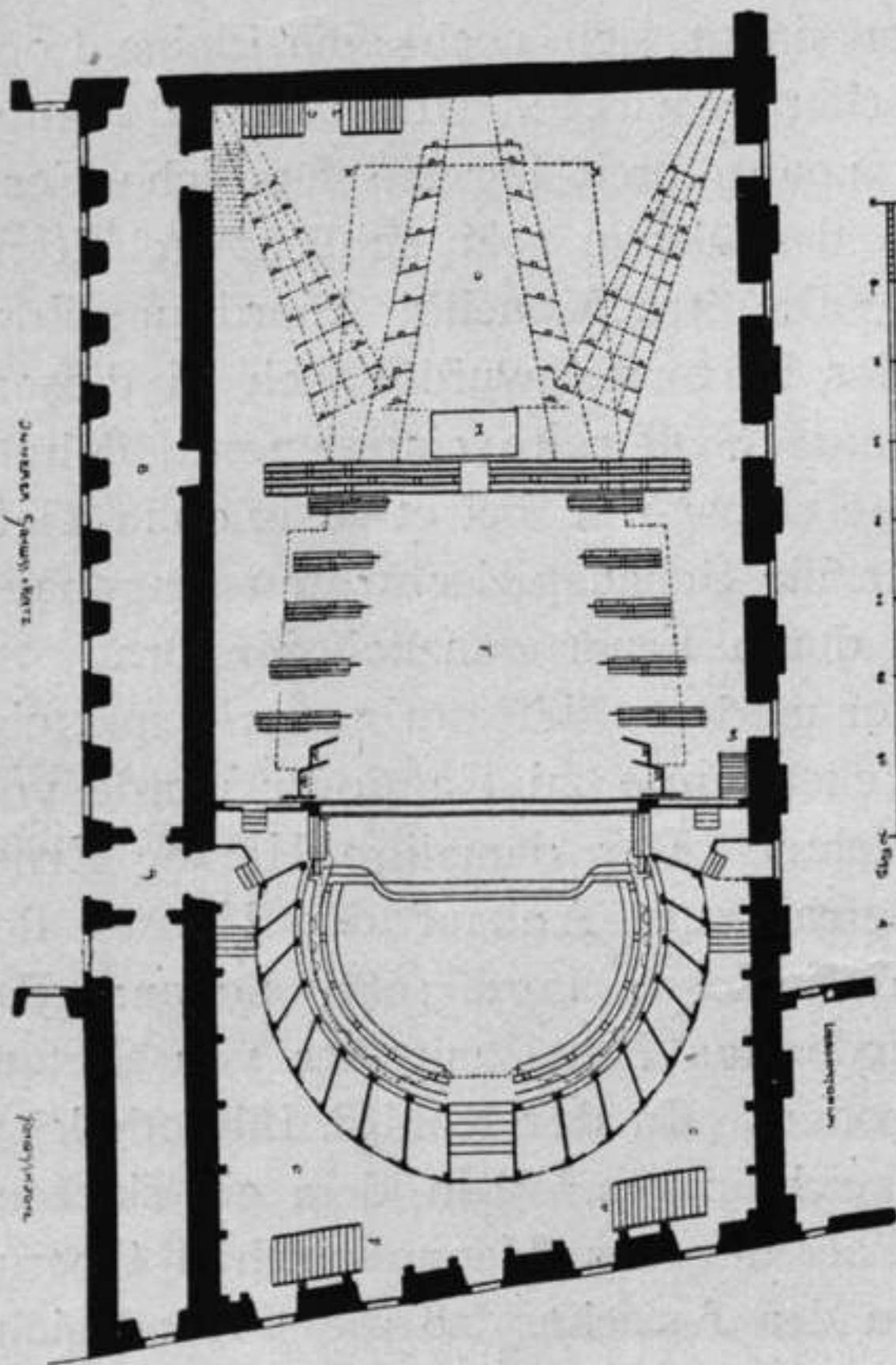
Fig. 89. Das hannoversche Opernhaus.
