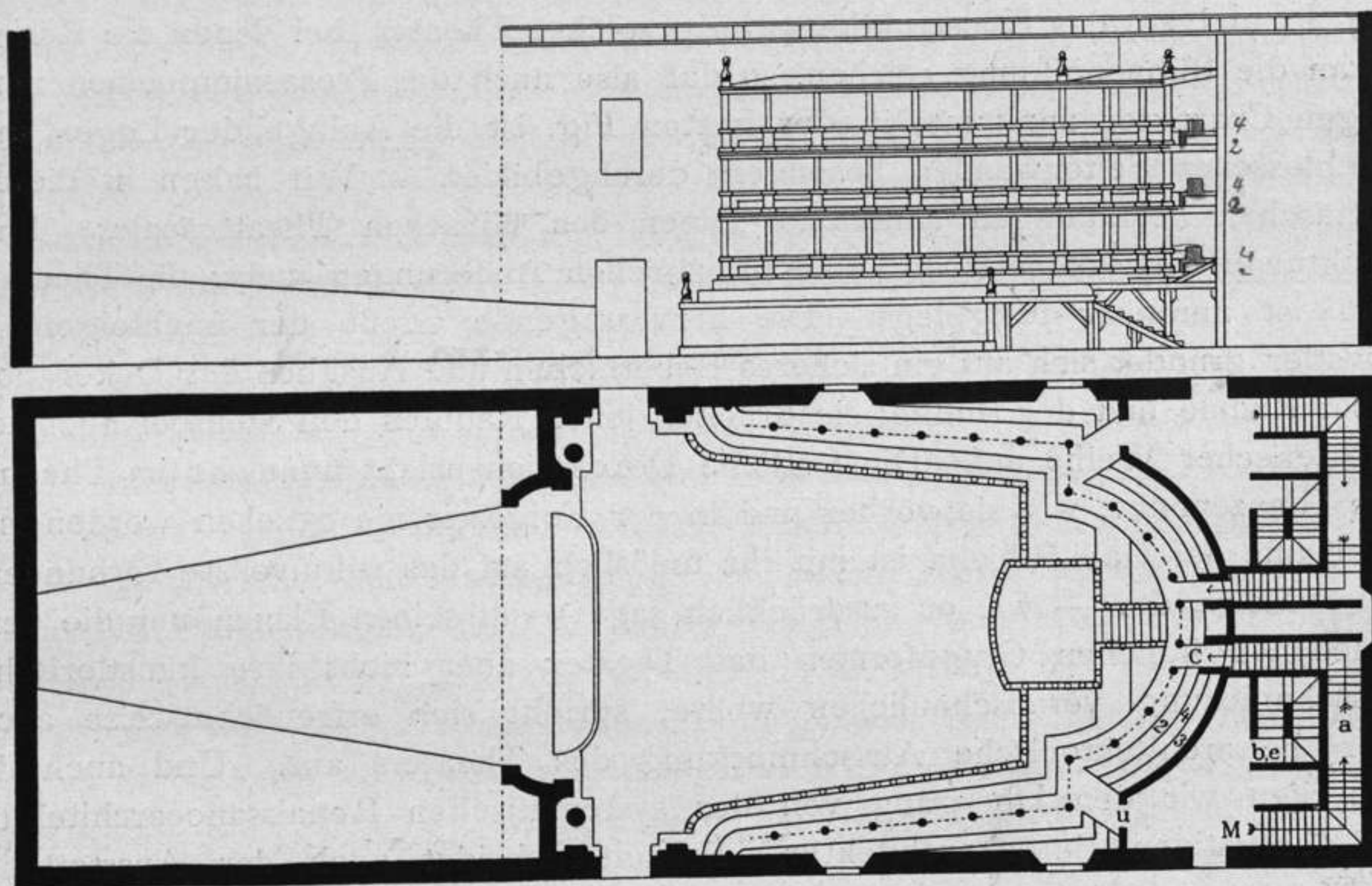
Fig. 21. Theatertypus nach Originalplänen Mottas.
