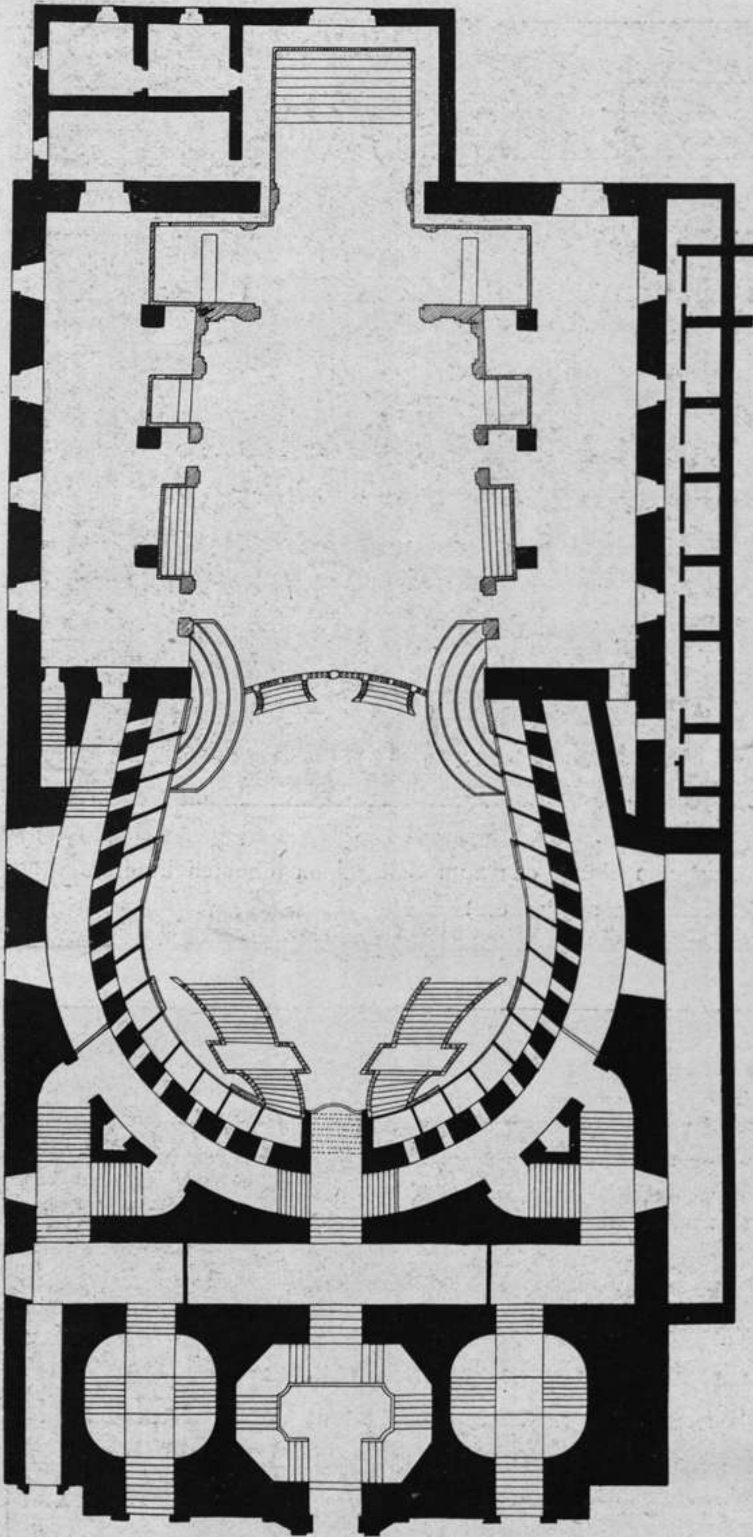
Fig. 54. Theater S. Carlo in Neapel: Grundriß.
