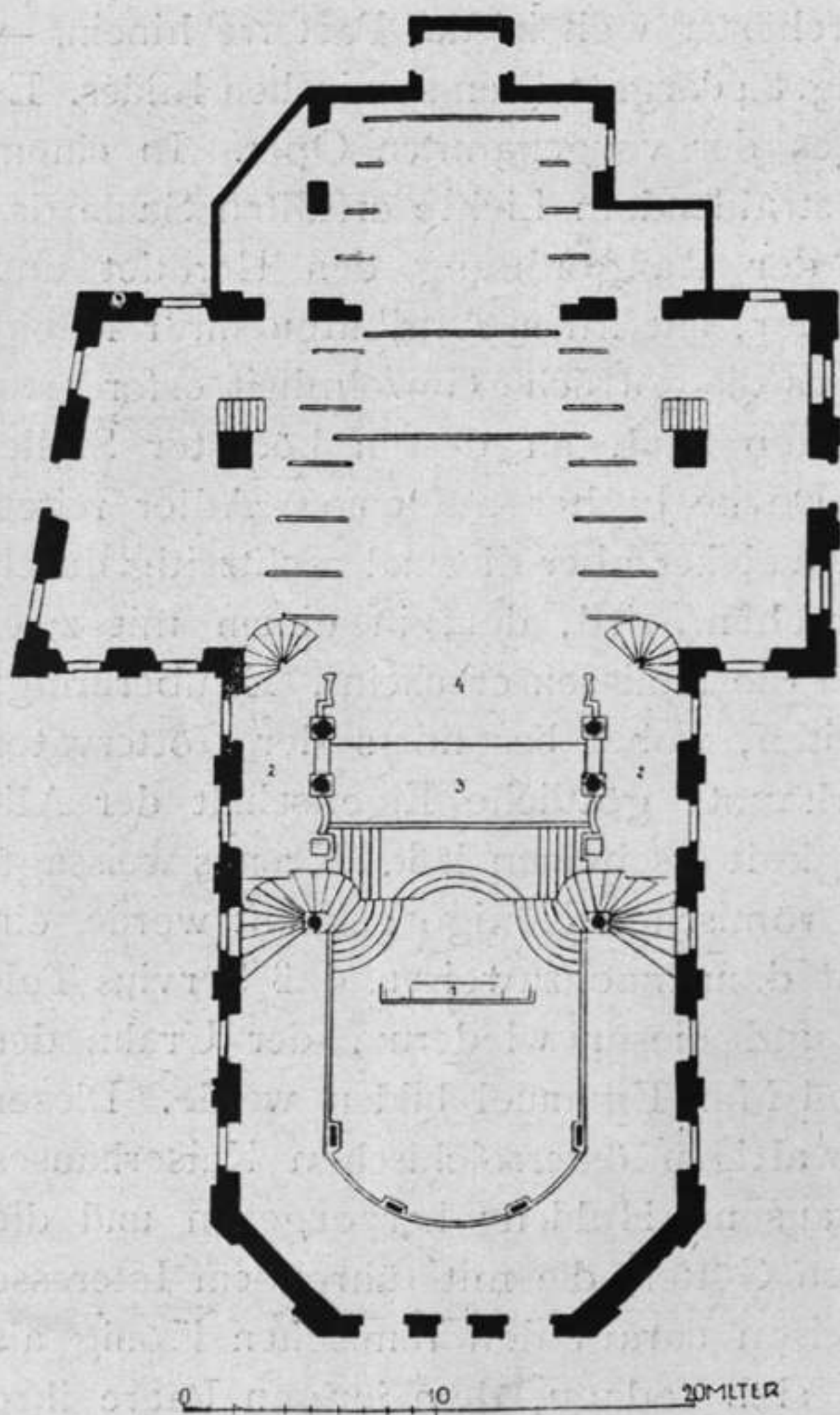
Fig. 85. Das erste Opernhaus zu Dresden. („Das Komödienhaus“.)
