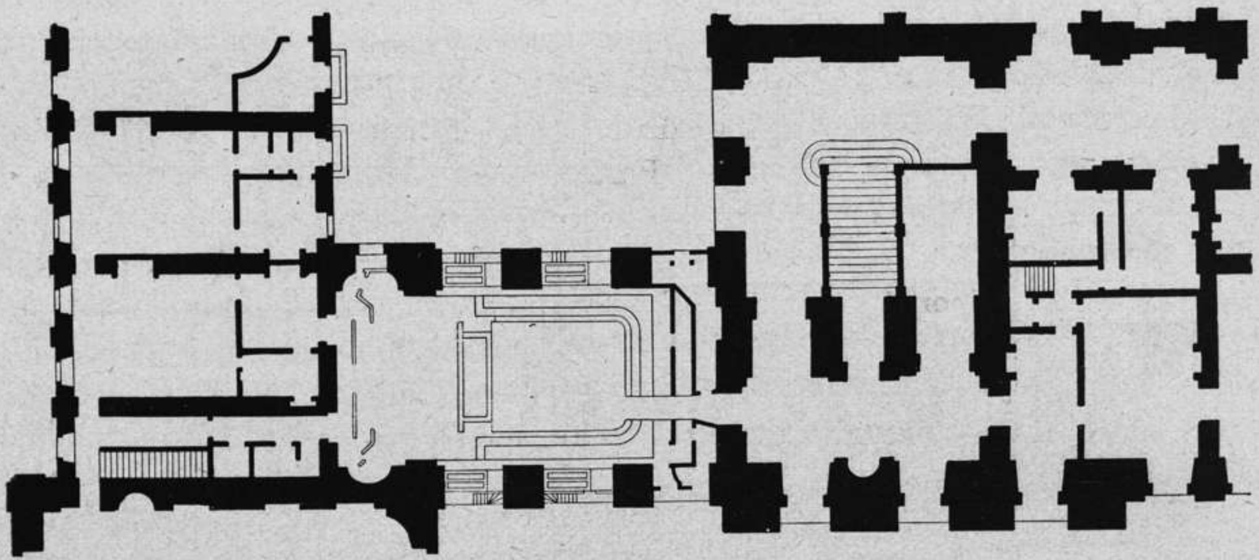
Fig. 45. Das kleine Schloßtheater zu Versailles.
