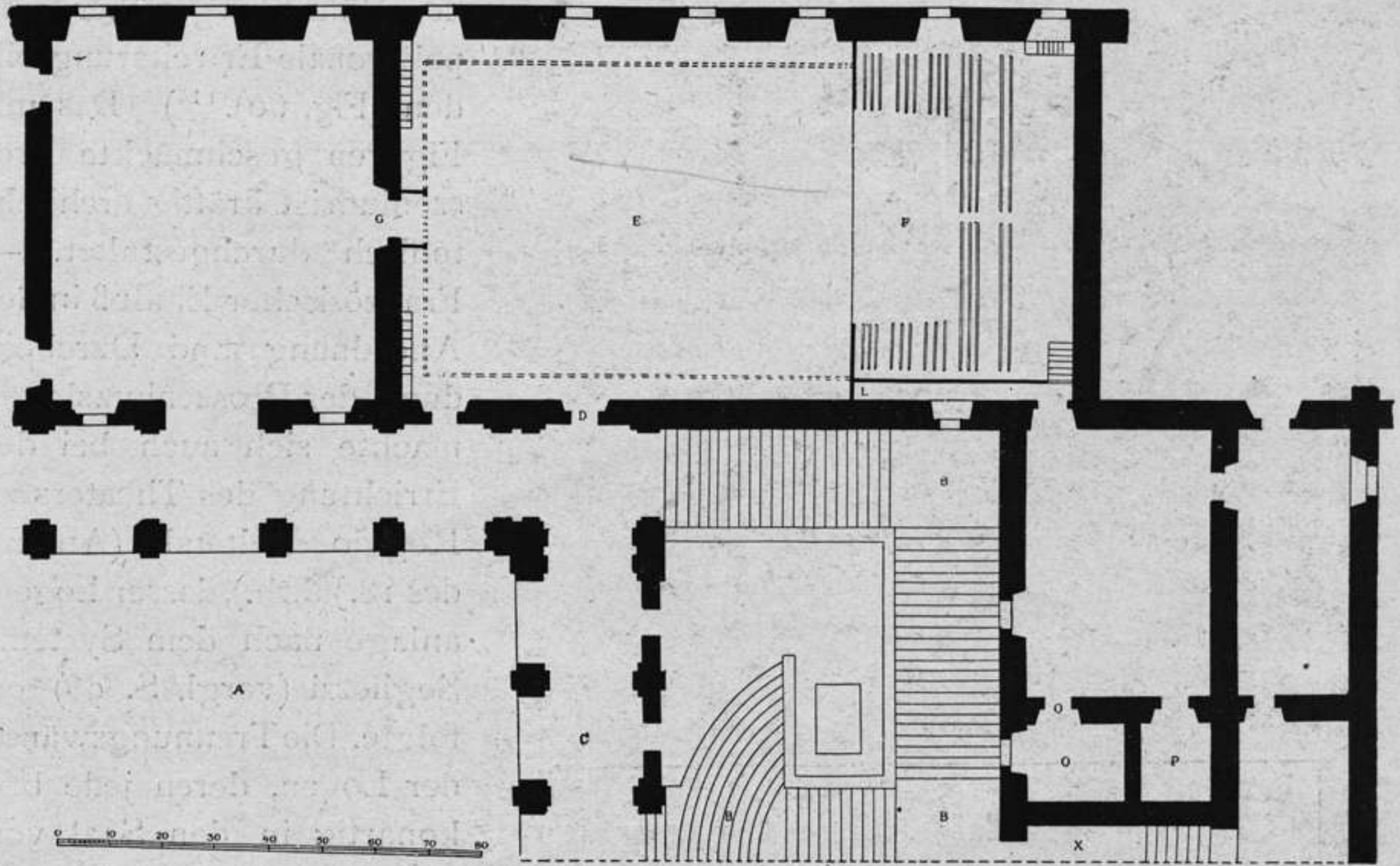
Fig. 58. Saaltheater im Palazzo reale zu Neapel.
