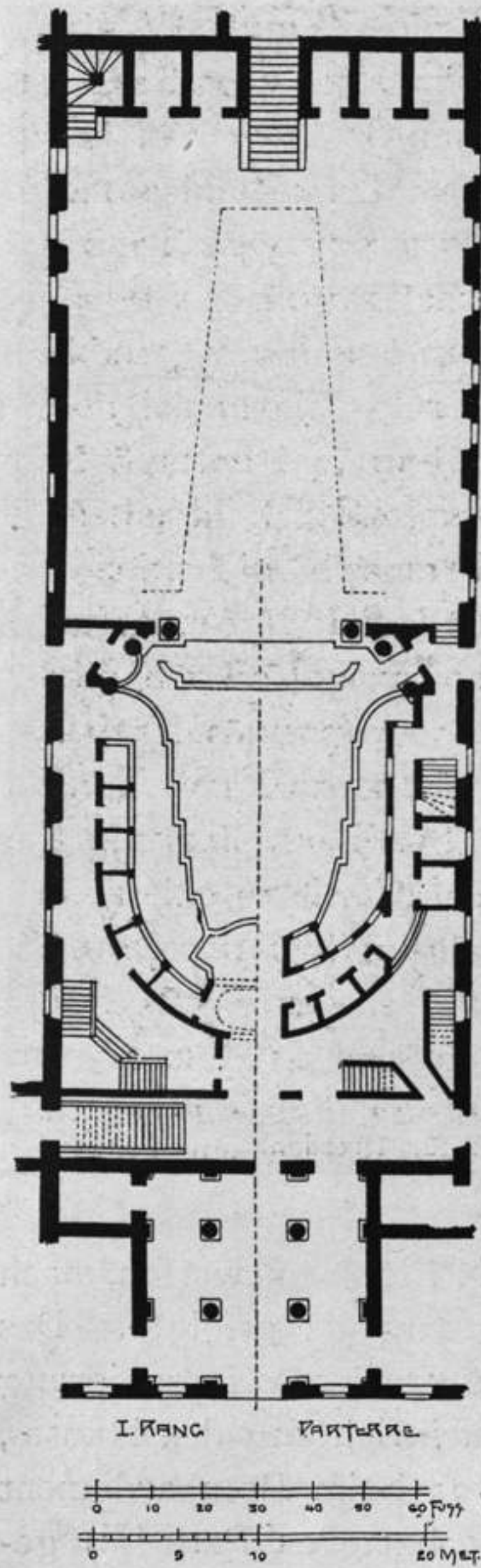
Fig. 103. Das Opernhaus in Mannheim.
