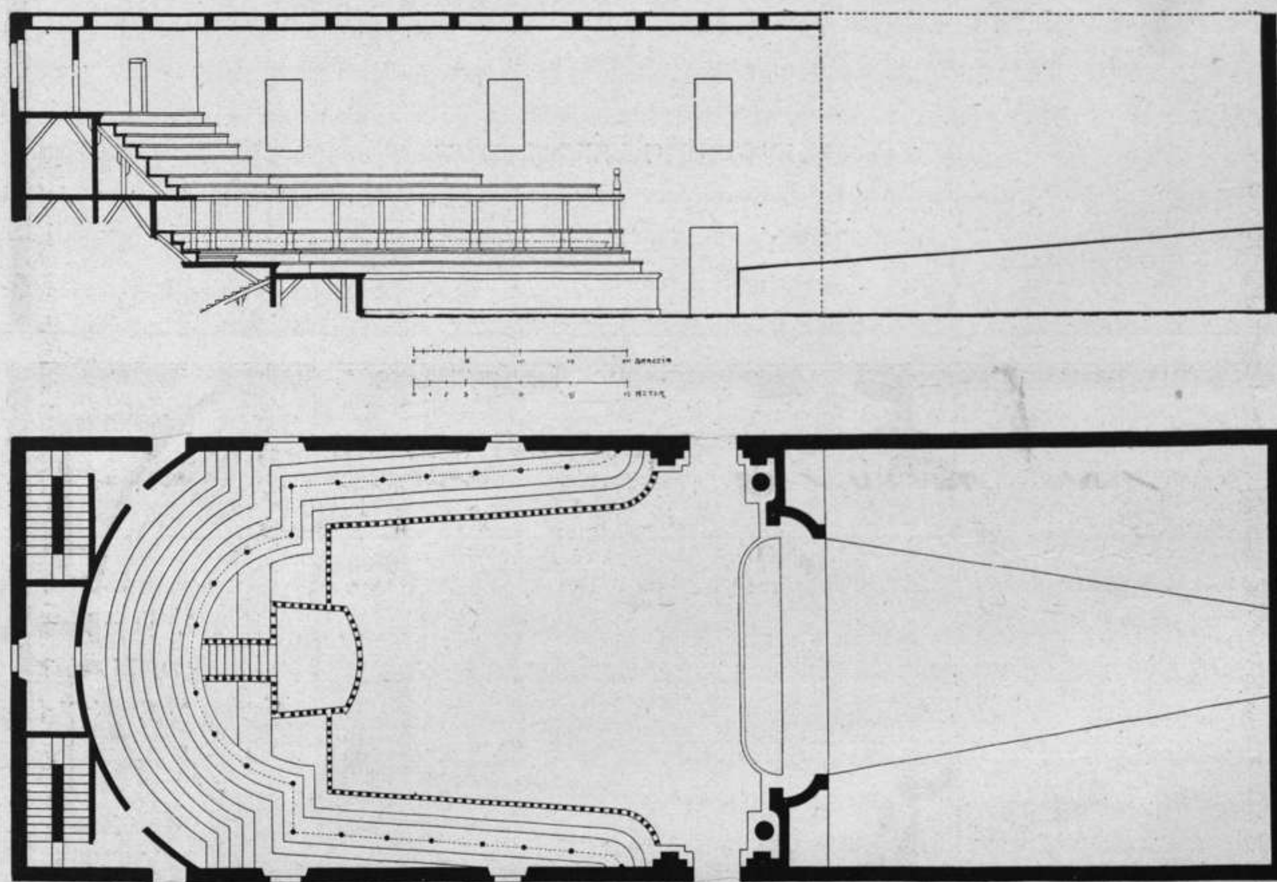
Fig. 20. Theatertypus nach Originalplänen Mottas.
