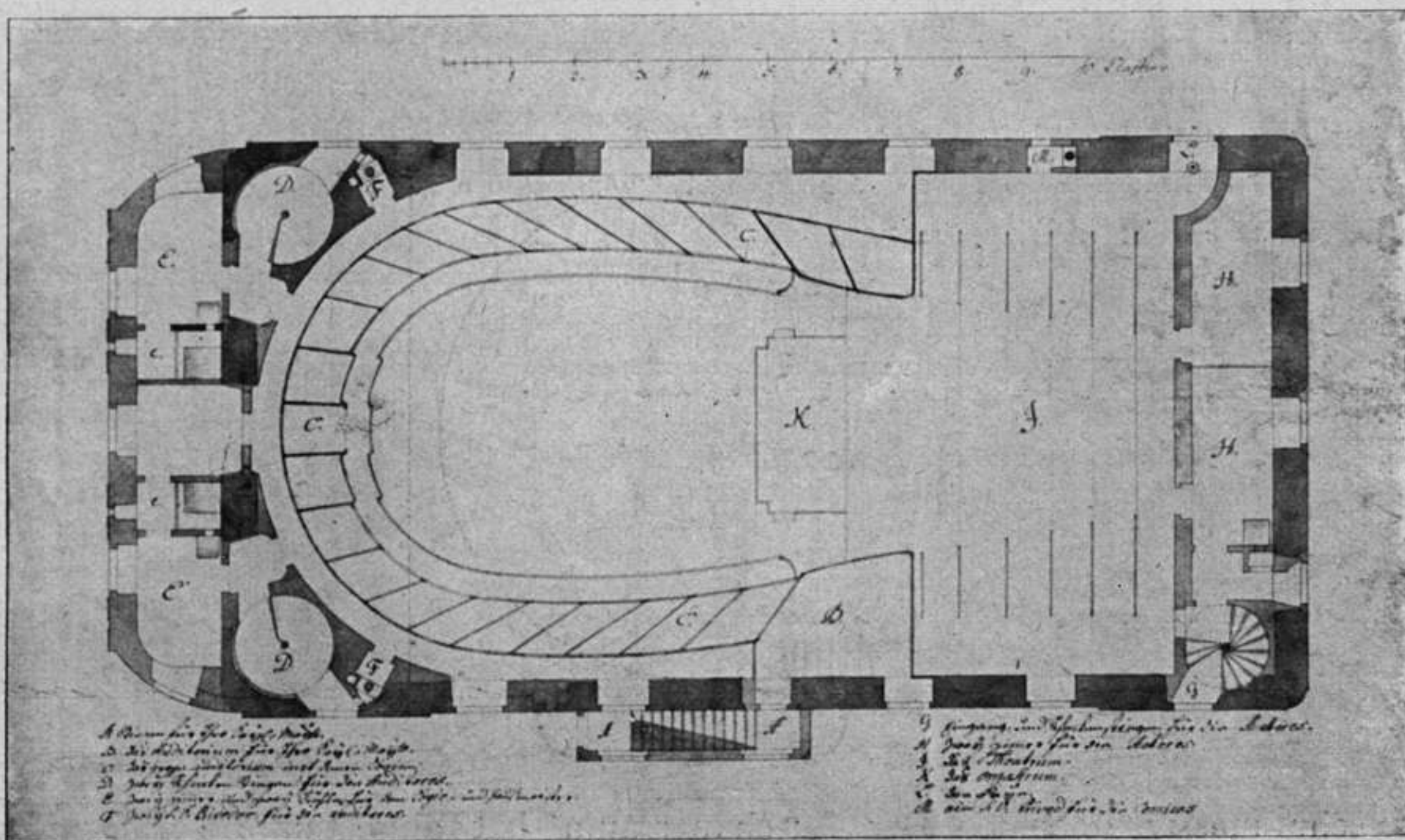
Fig. 132. Hofburgtheater in Wien bis 1756.
