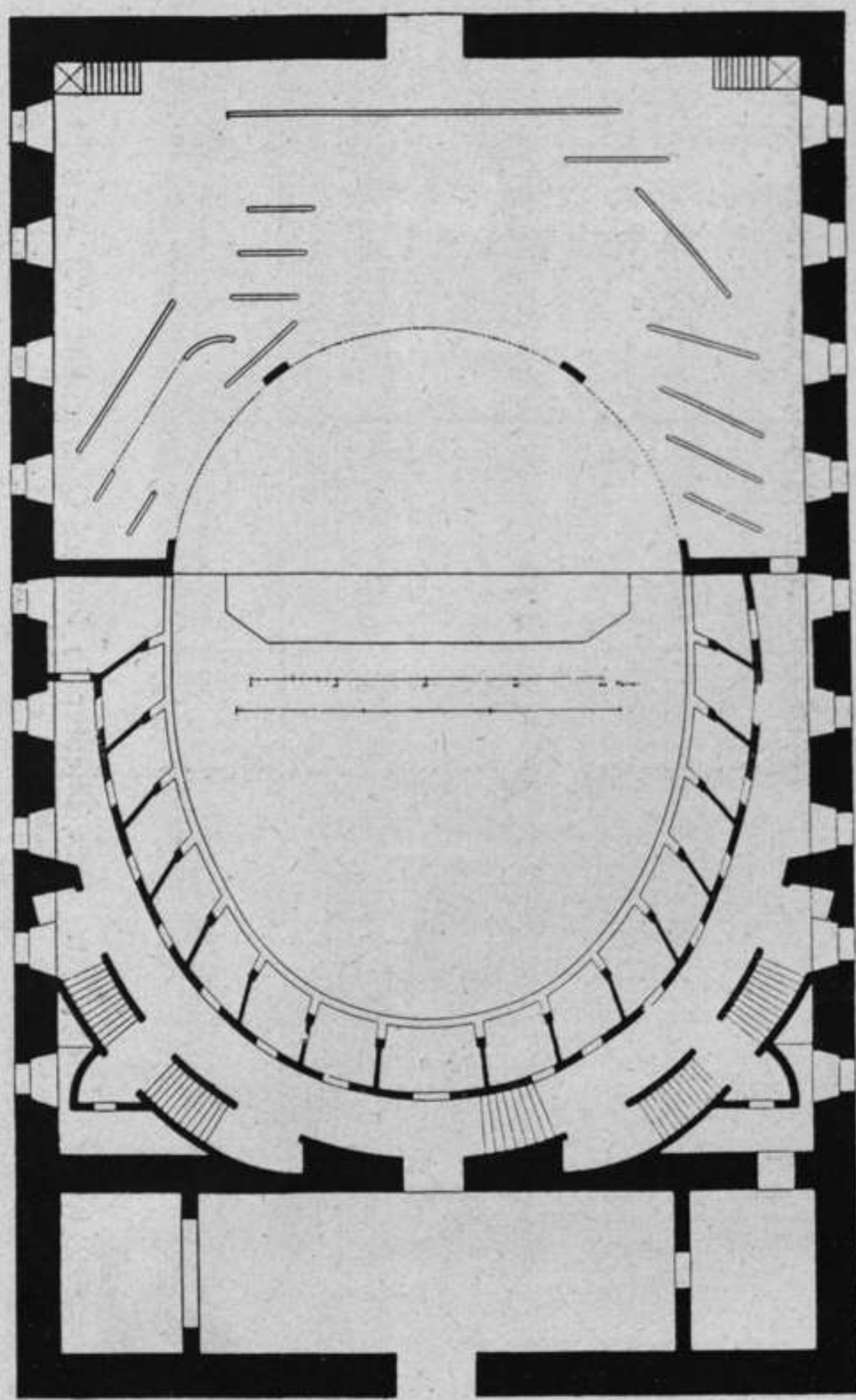
Fig. 74. Das Theater zu Imola.
