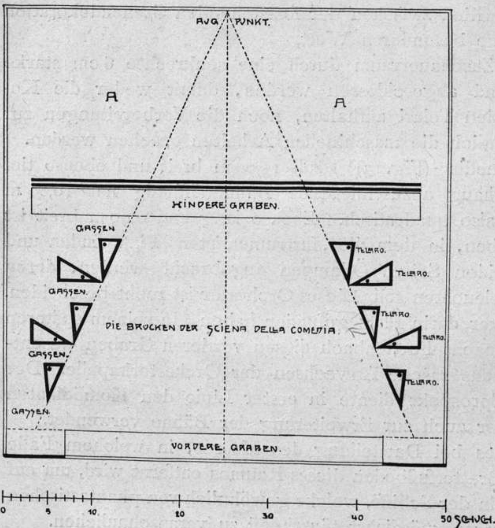
Fig. 13. Die Telaribühne. (Nach Joseph Furtenbach.)
