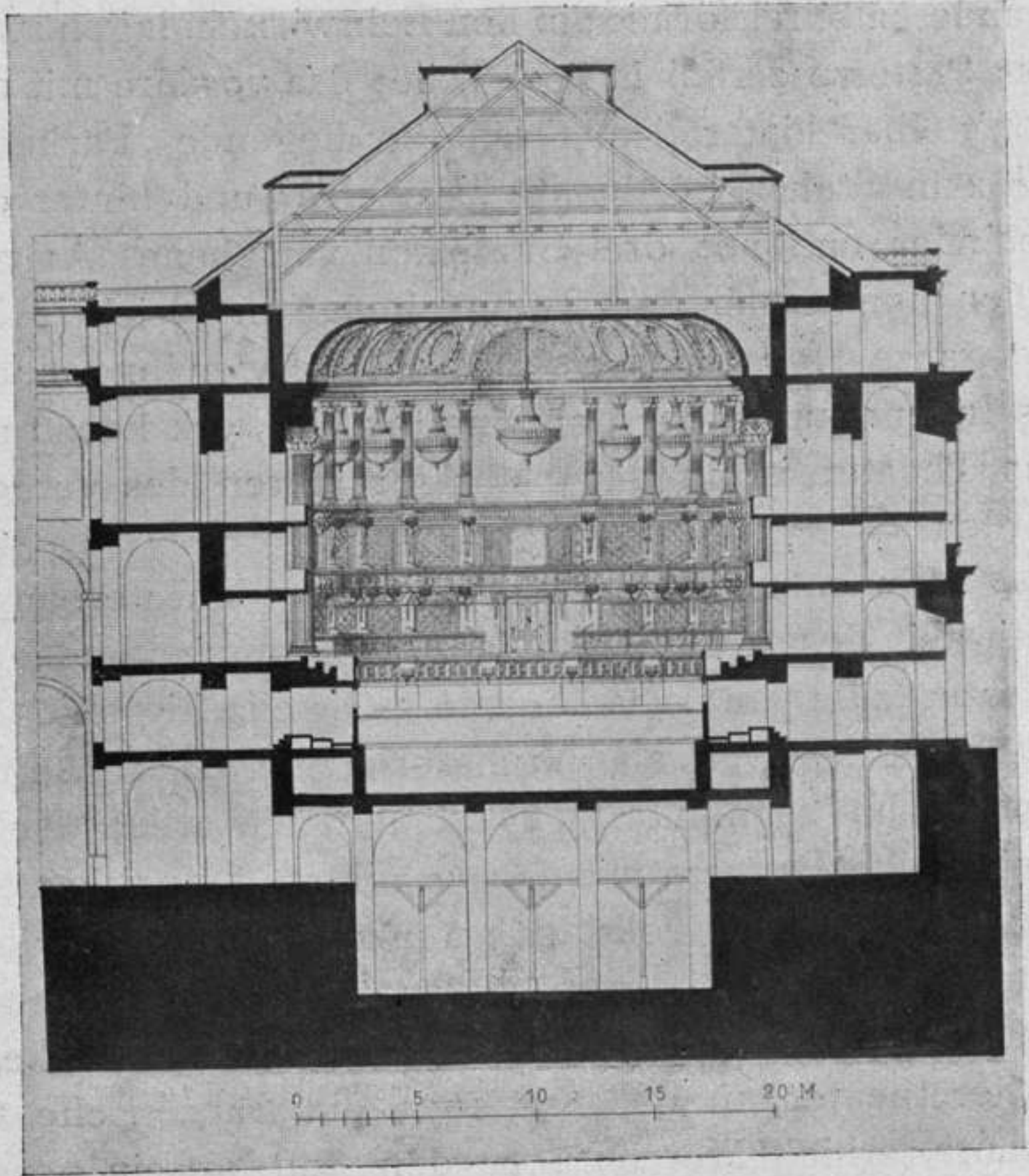
Fig. 48. Das Opernhaus zu Versailles: Querschnitt.
