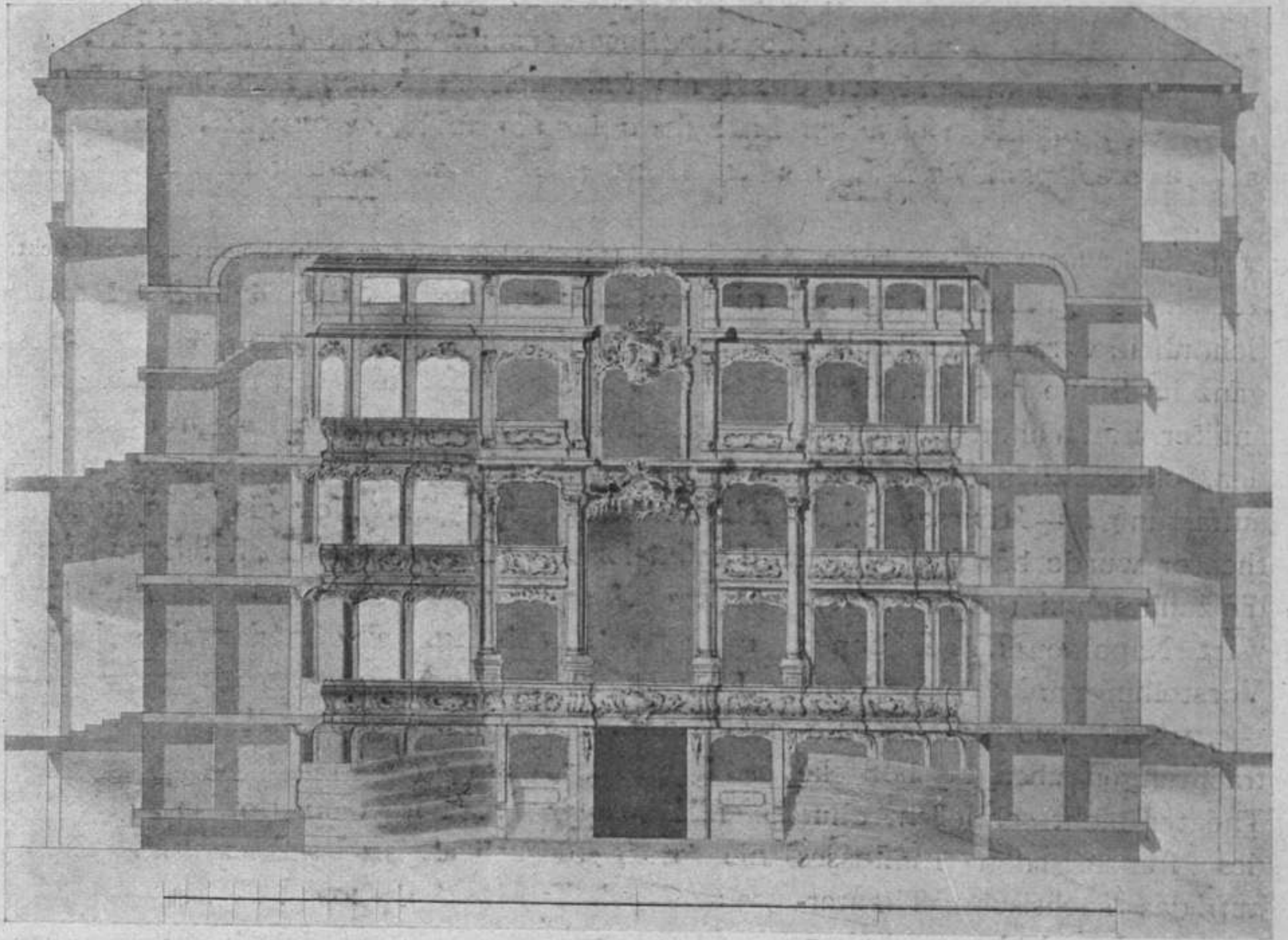
Fig. 137. Umbauprojekt für das Opernhaus zu Dresden. (2. Hälfte des 18. Jahrhunderts.)
