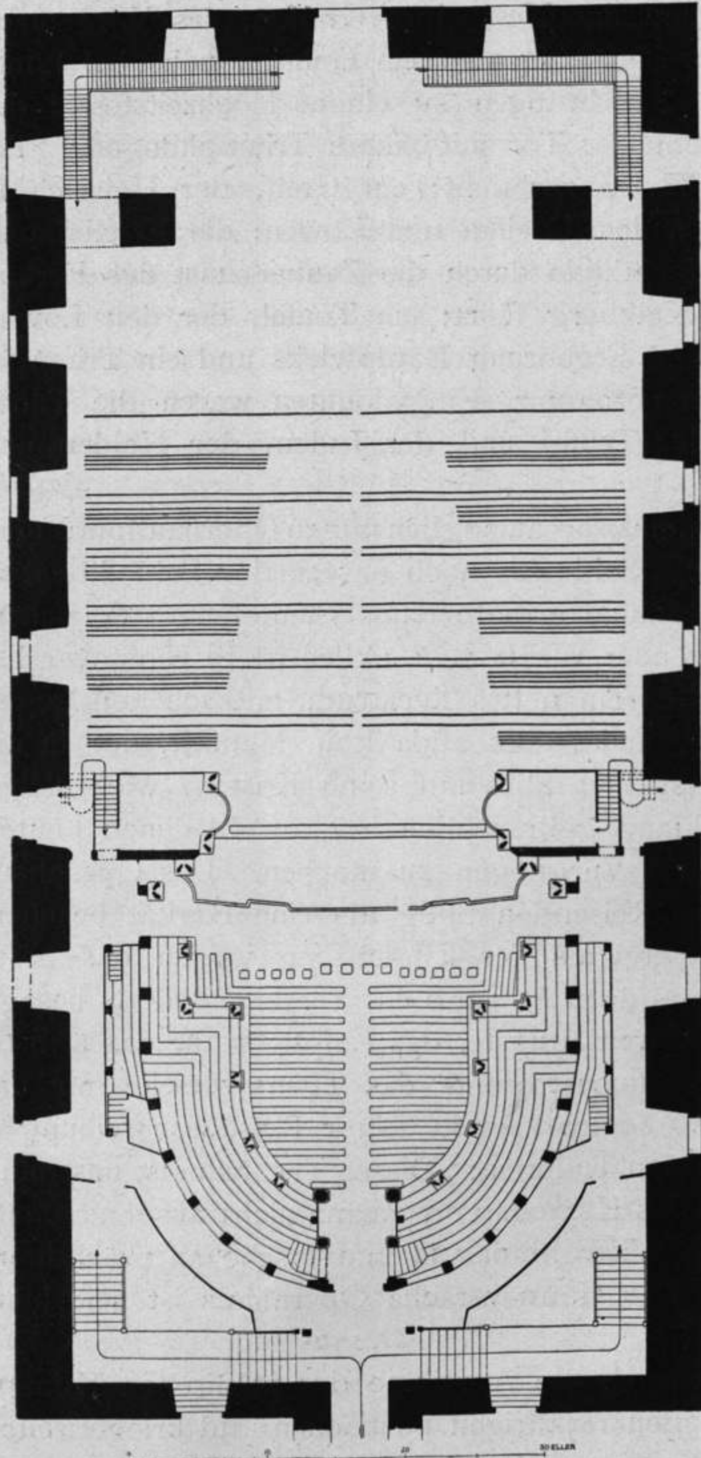
Fig. 91. Das große Opernhaus in Dresden von Alessandro Mauro (1718—1719 erbaut).
