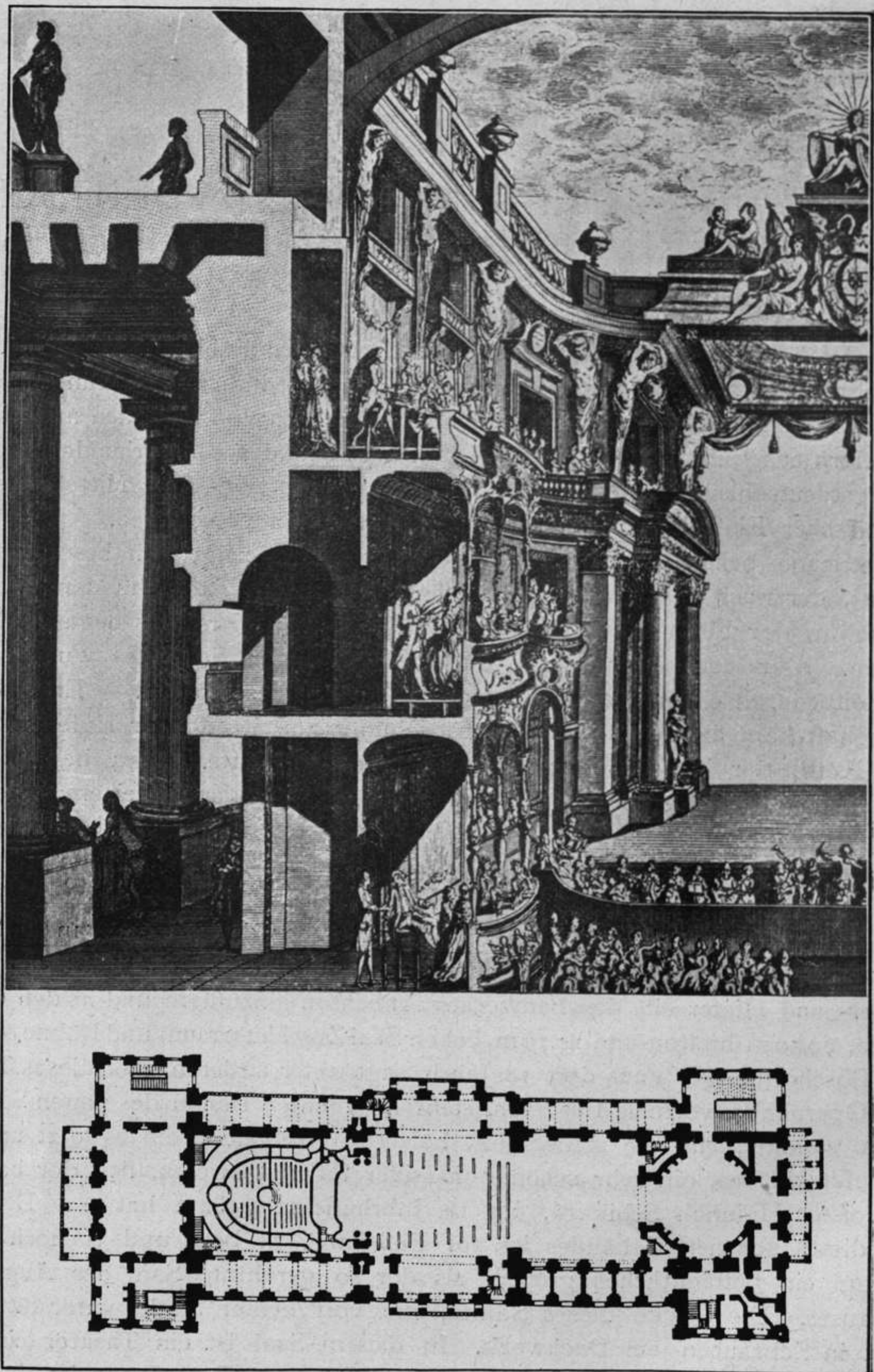
Fig. 123. Stuttgarter Opernhaus. (Nach einem Originalplane des Louis Philipp de la Guepière.)
