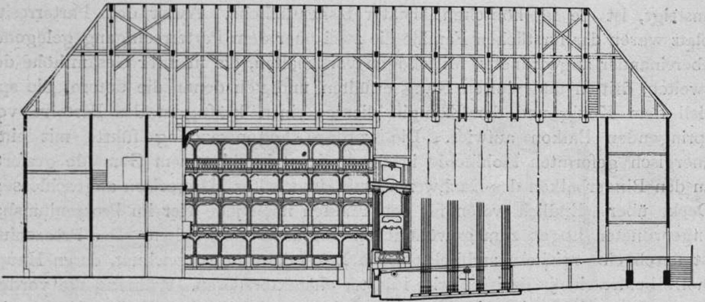
Fig. 111. Das Opernhaus in Warschau.
