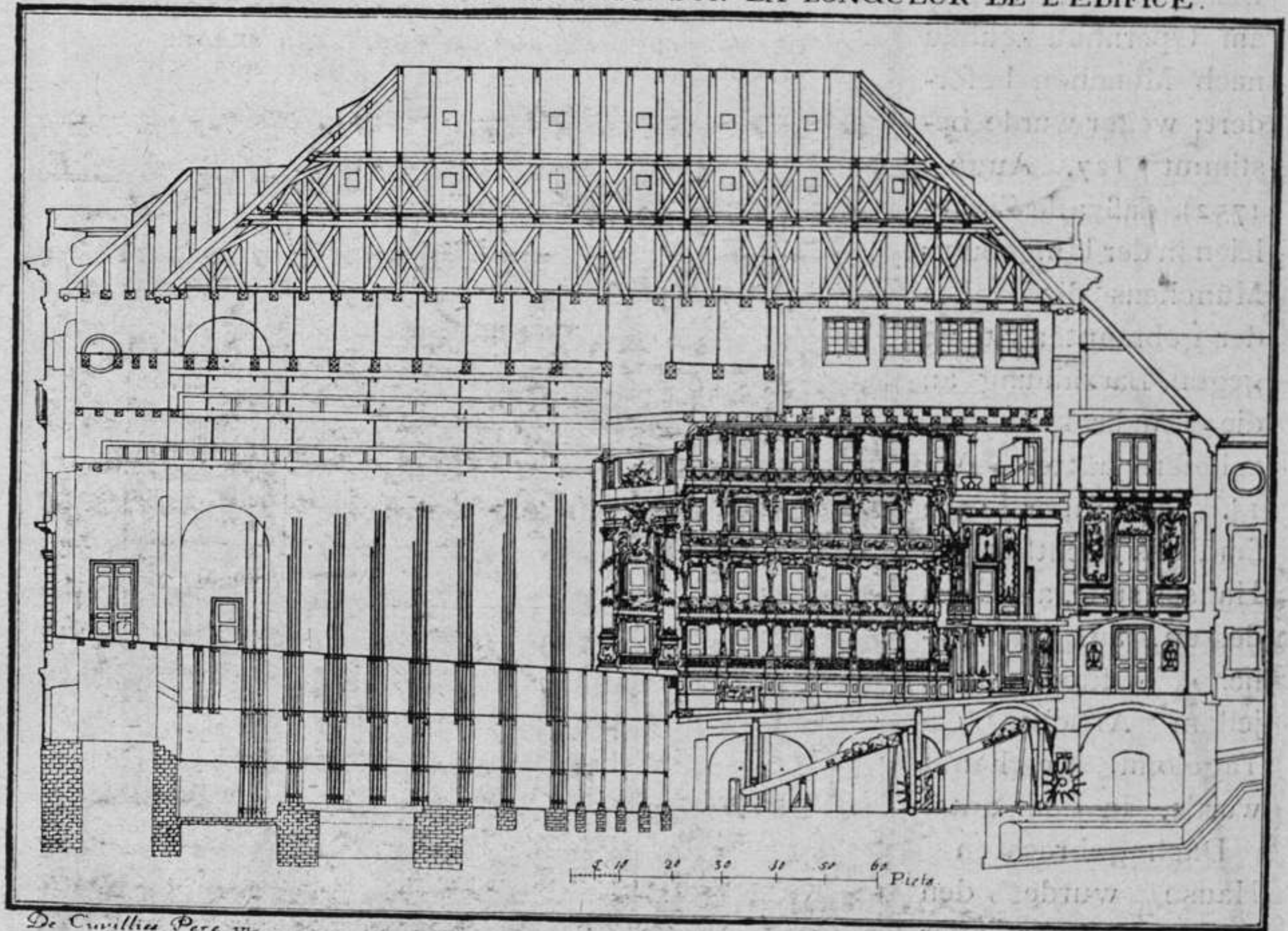
Fig. 127. Längenschnitt durch das Opernhaus (jetzt kgl. Residenztheater).
