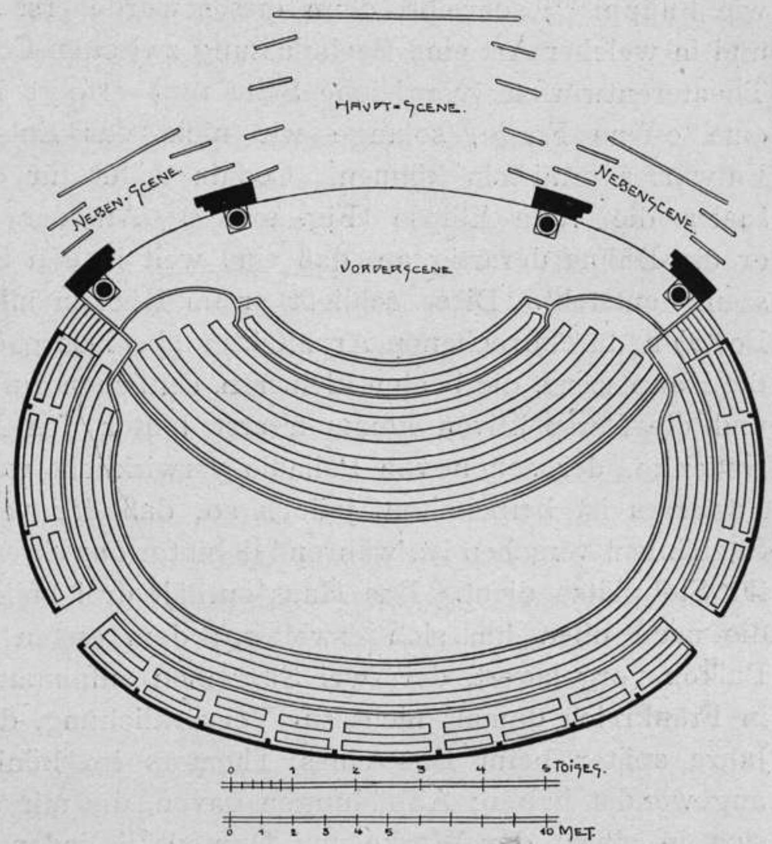
Fig. 49. Theaterprojekt von Cochin.
