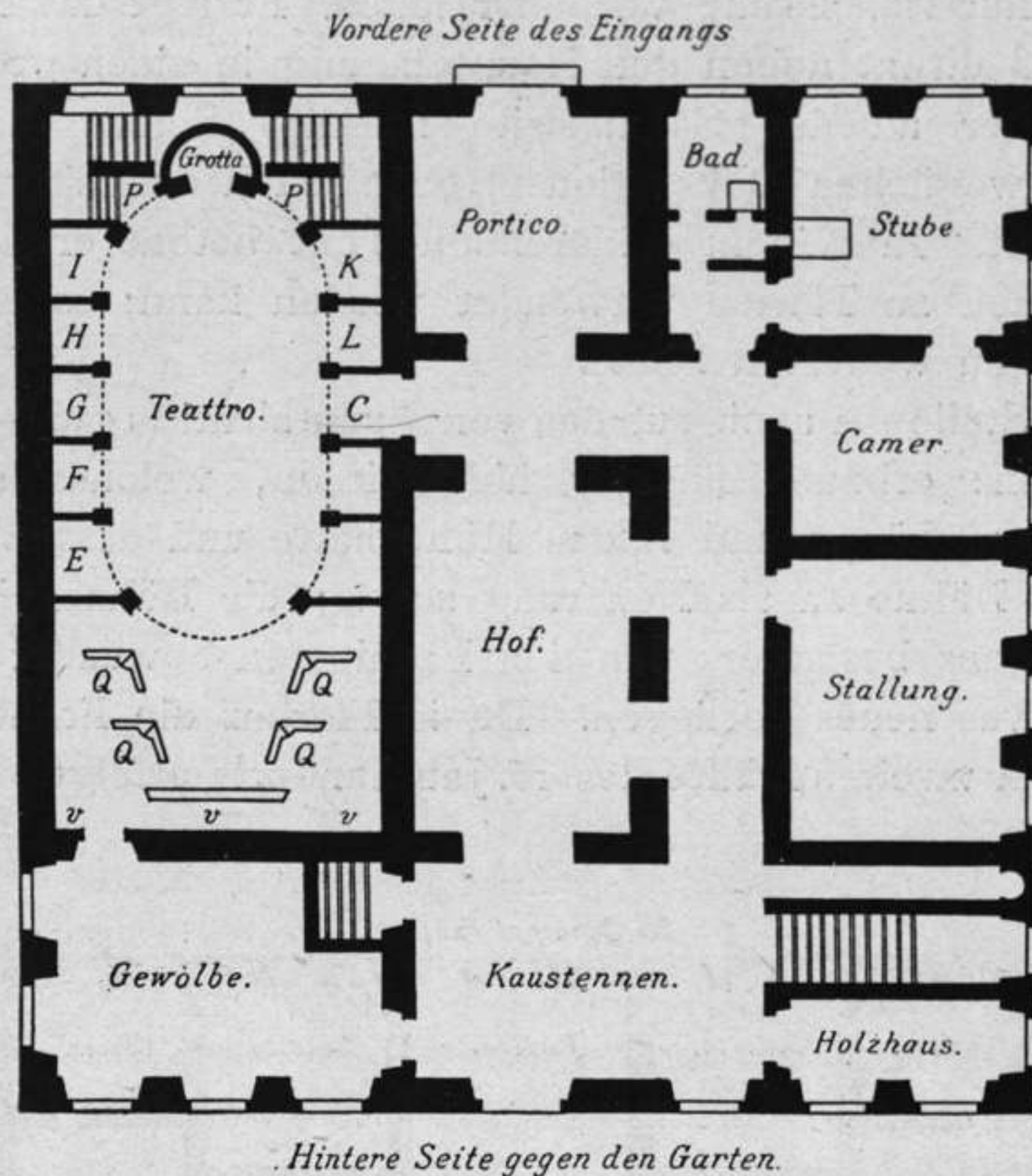
Fig. 12. Haustheater nach einem Projekte Furttentbachs.
