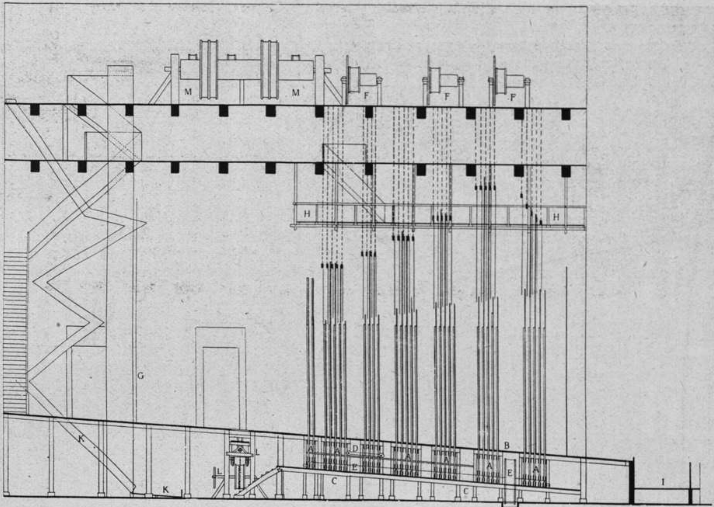
Fig. 116. Das Dresdner Opernhaus 1749: Bühneneinrichtung.
