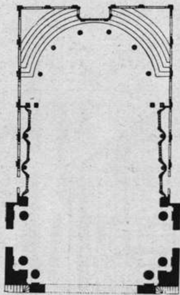
Fig. 40. Salle des machines: 1. Rang.
