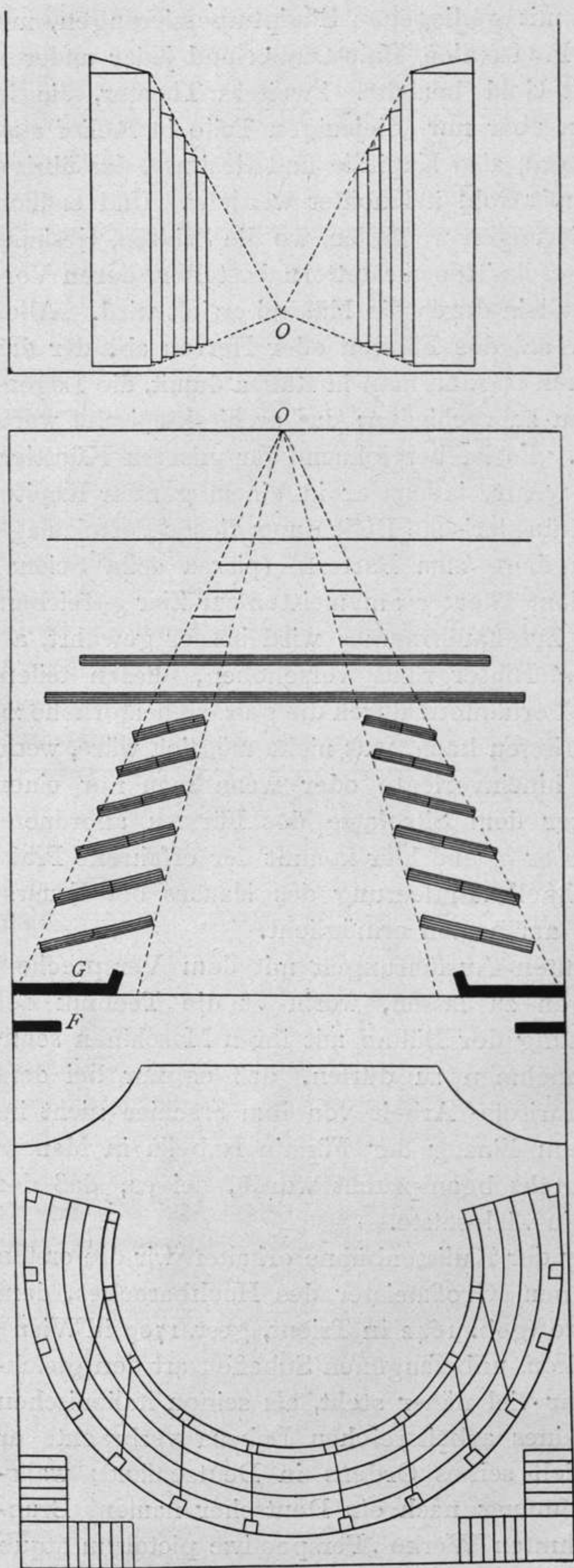
Fig. 24. Theaterprojekt des Pozzo.
