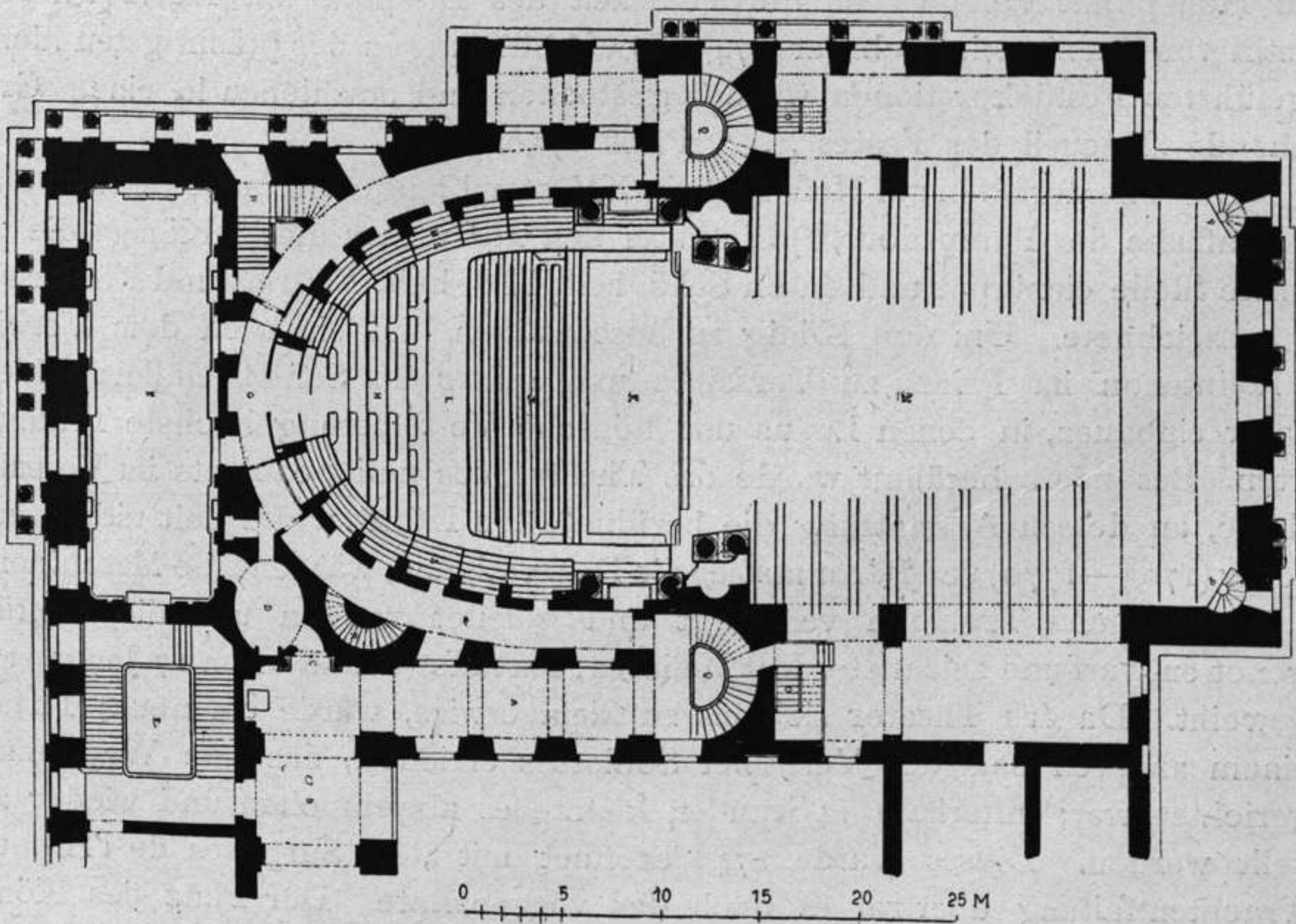
Fig. 47. Das Opernhaus zu Versailles: Grundriß.
