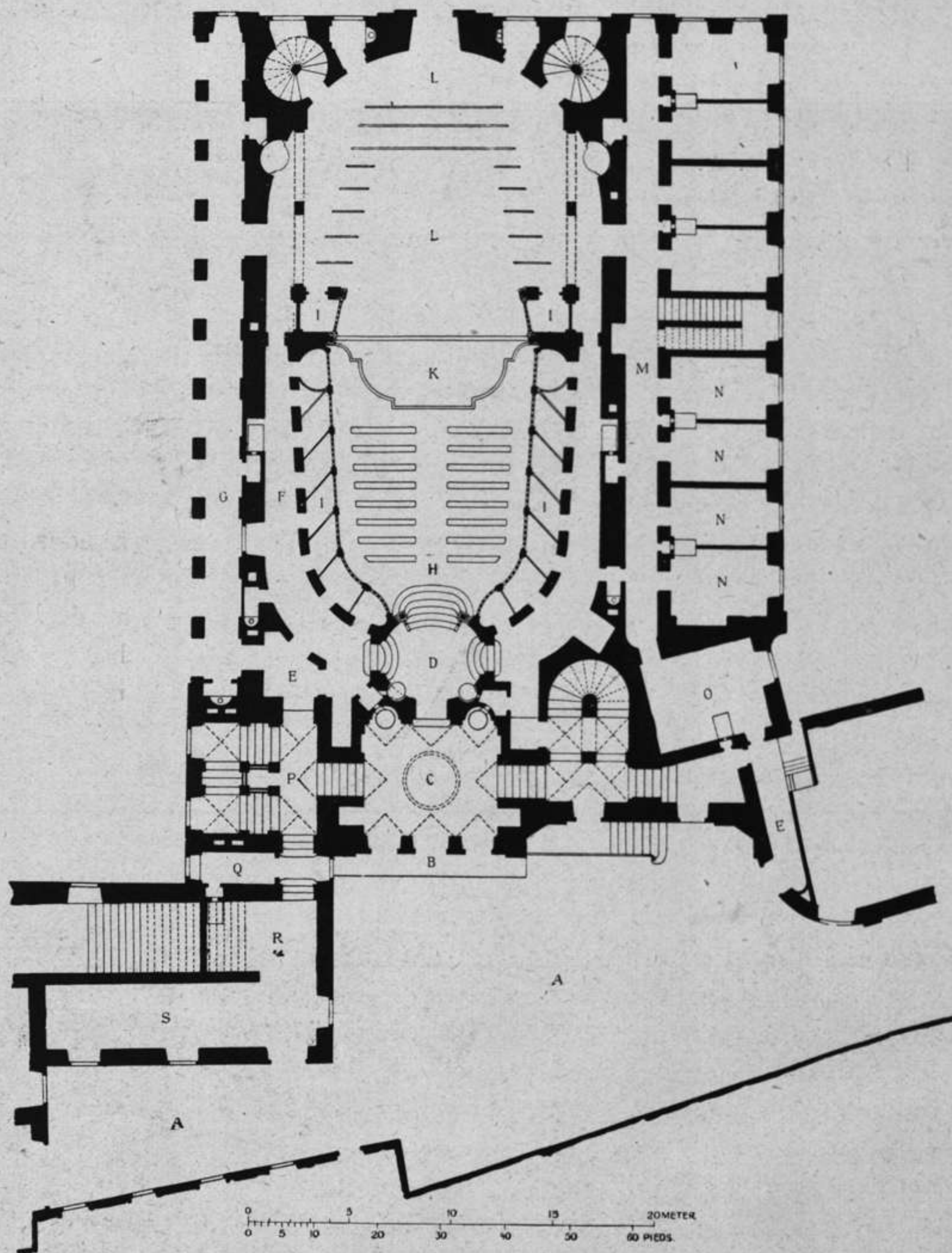
Fig. 129. Das königliche Residenztheater in München.
