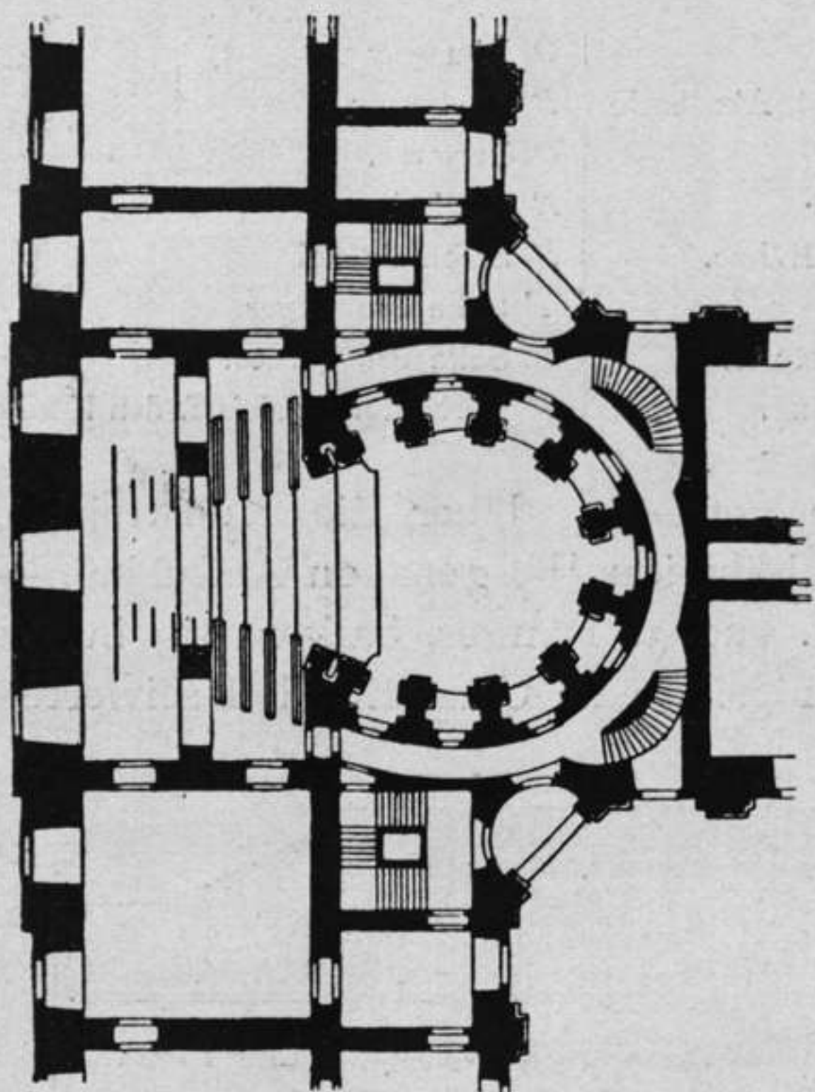
Fig. 67. Schloßtheater zu Caserta: Grundriß.
