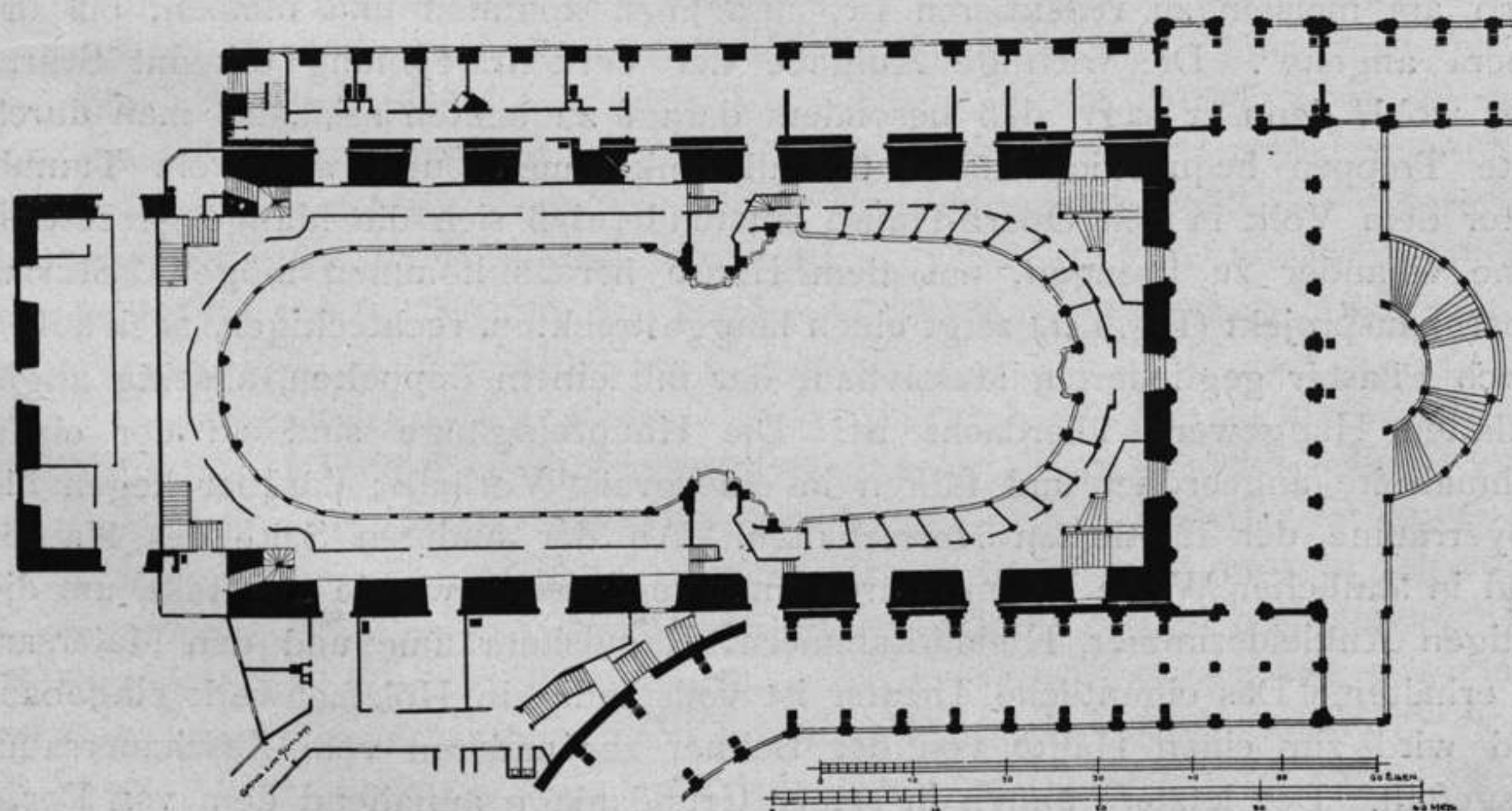
Fig. 140. Das Dresdner Opernhaus als Redoutensaal. (Umgebaut 1772.)
