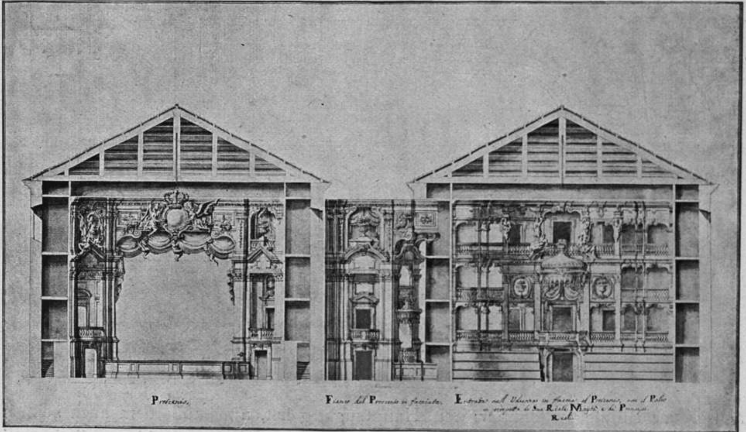
Fig. 118. Theaterentwurf des Giuseppe Galli-Bibiena in Dresden.
