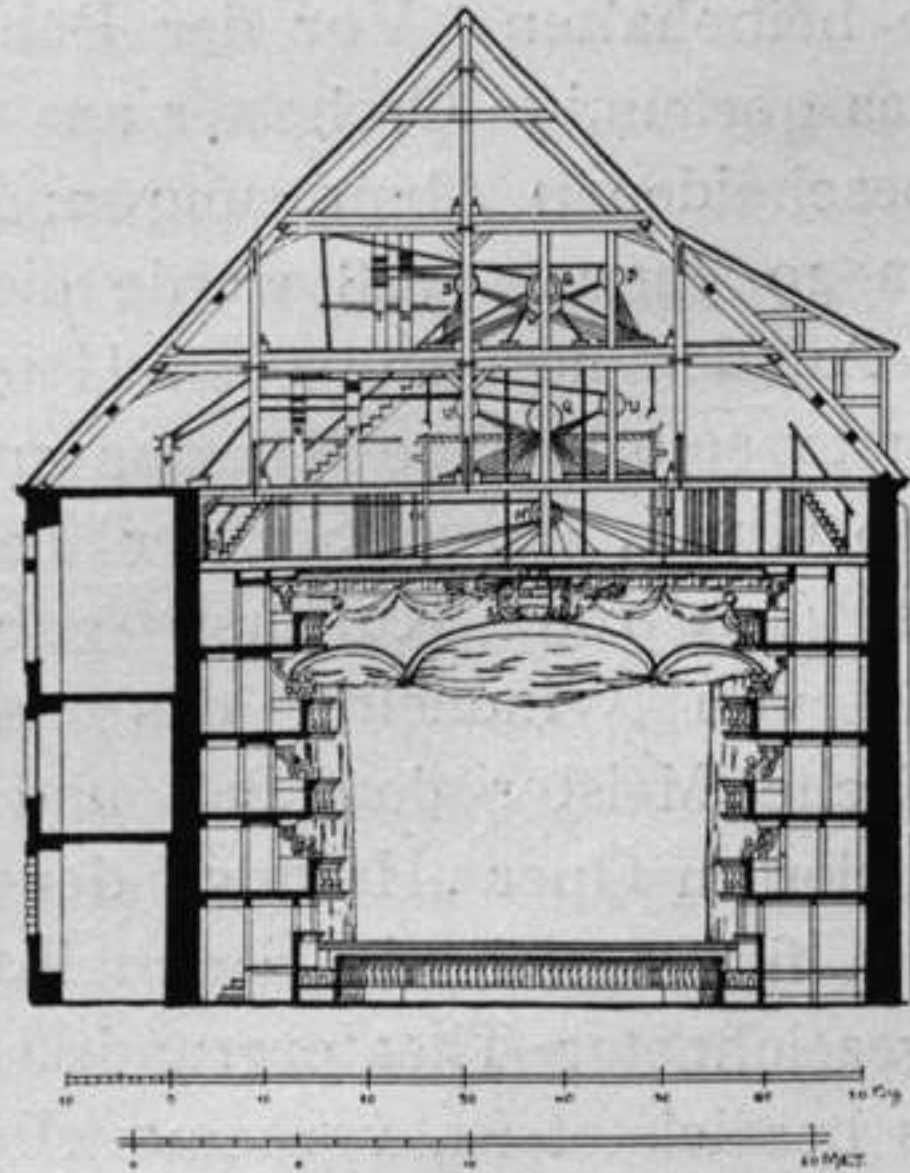
Fig. 90. Das hannoversche Opernhaus: Querschnitt.
