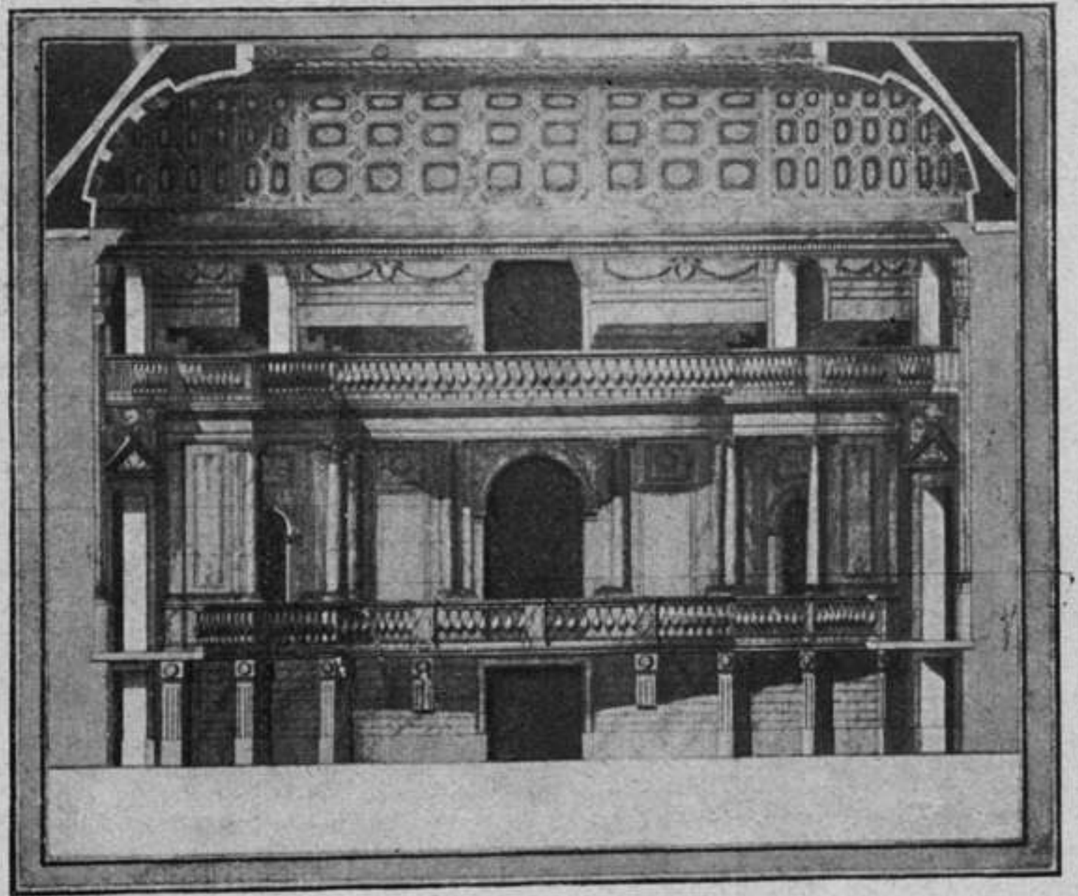
Fig. 136. Schloßtheater zu Schönbrunn: Kaiserl. Hofloge.
