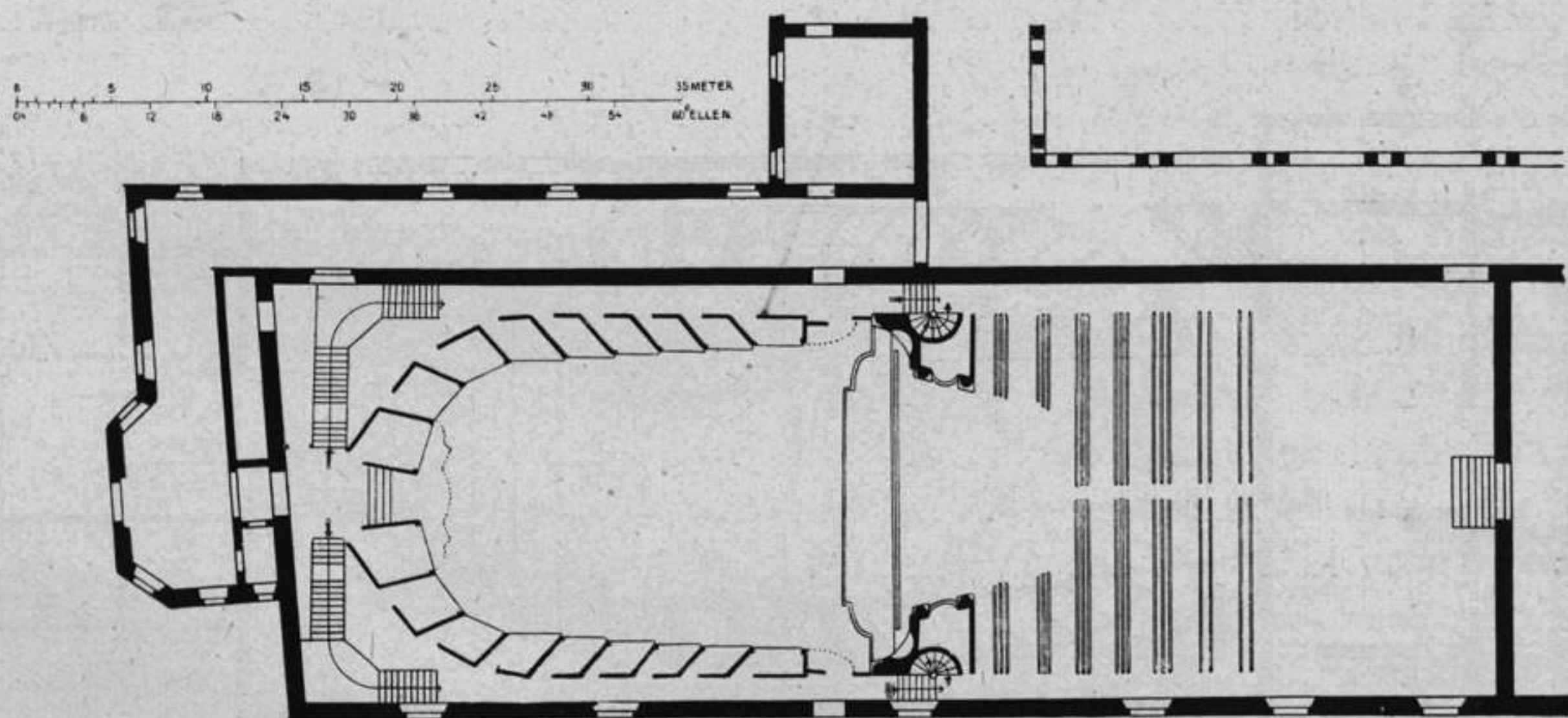
Fig. 70. Theater in Mantua.
