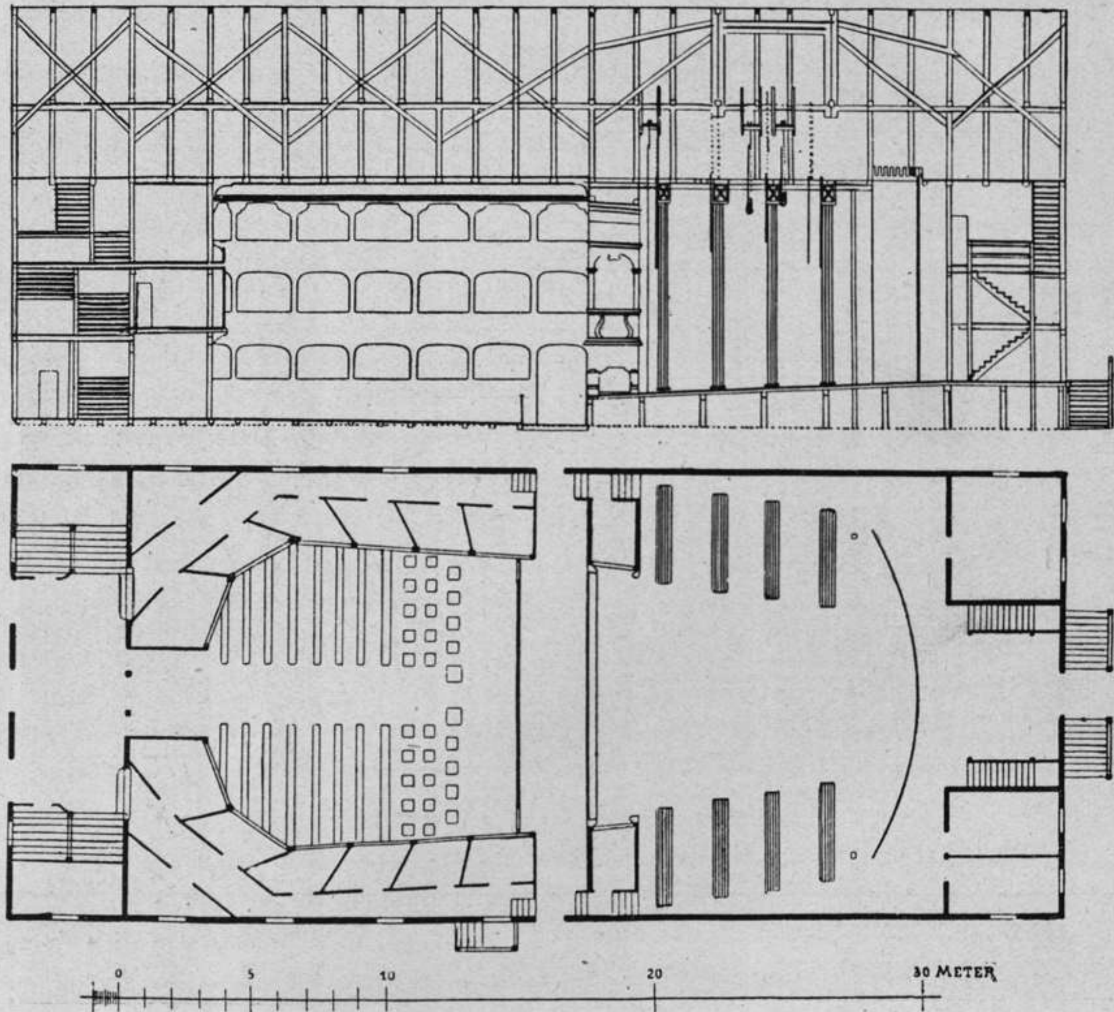
Fig. 87. Das „kleine Komödienhaus“ in Dresden.
