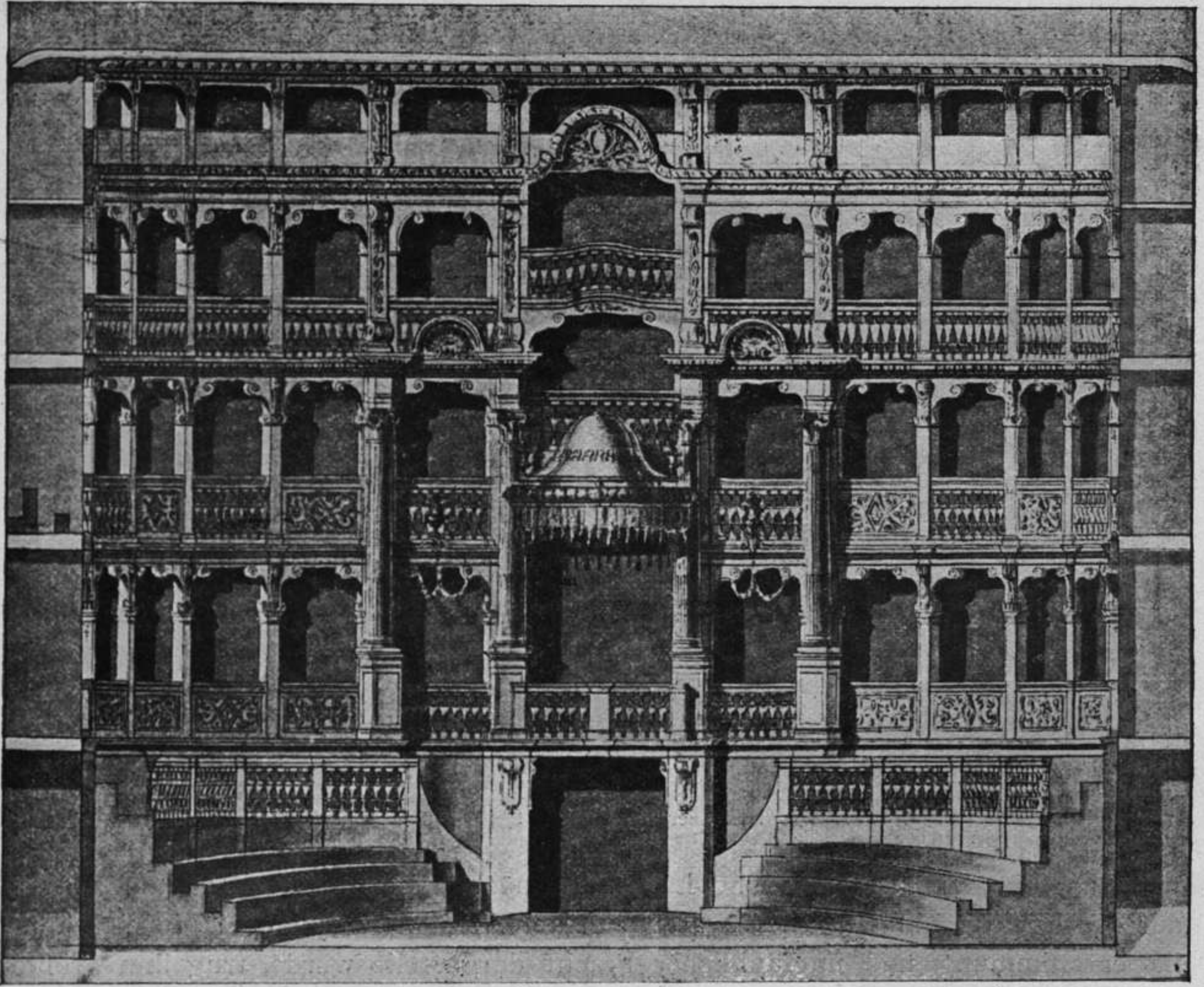
Fig. 115. Das Dresdner Opernhaus 1749: Ansicht der fürstlichen Mittelloge.
