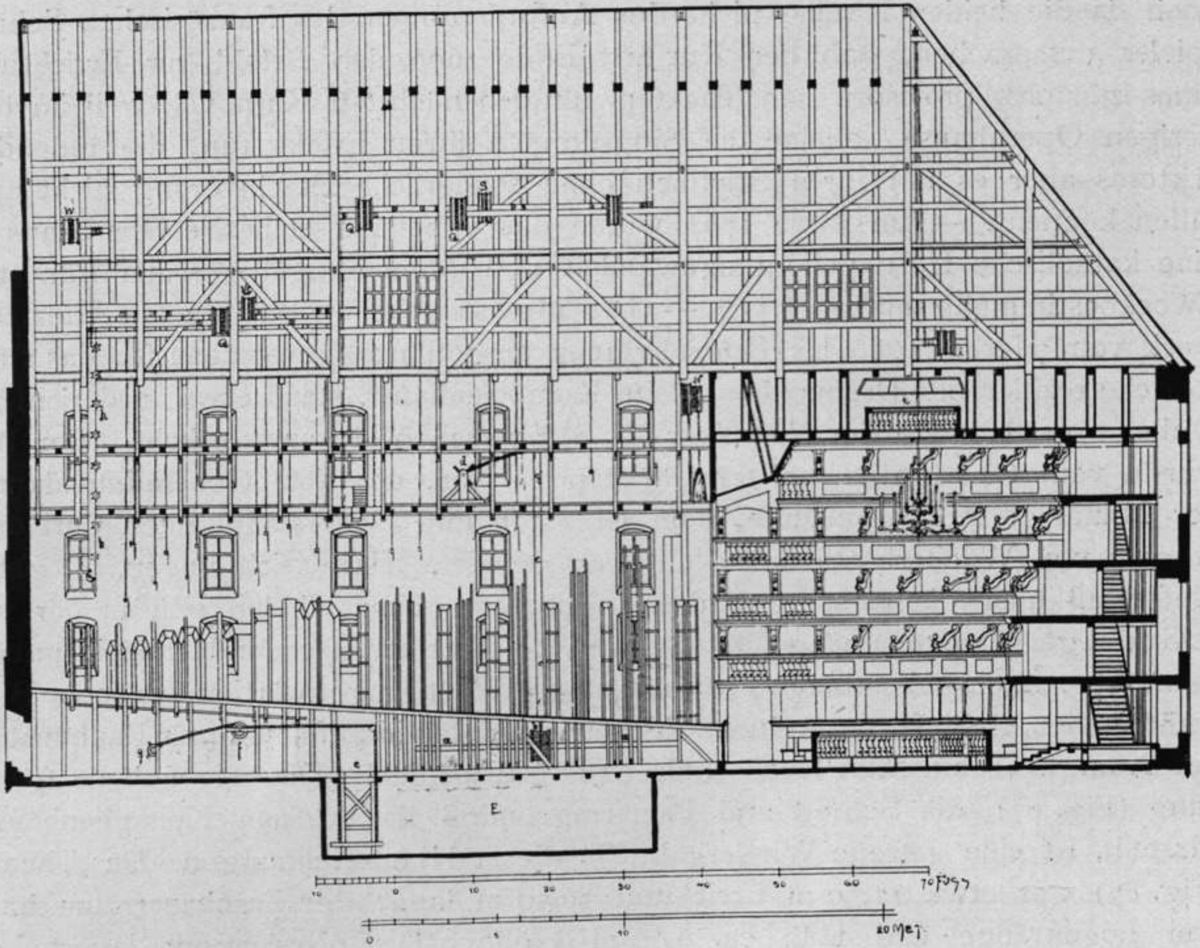
Fig. 88. Das hannoversche Opernhaus: Längenschnitt.
