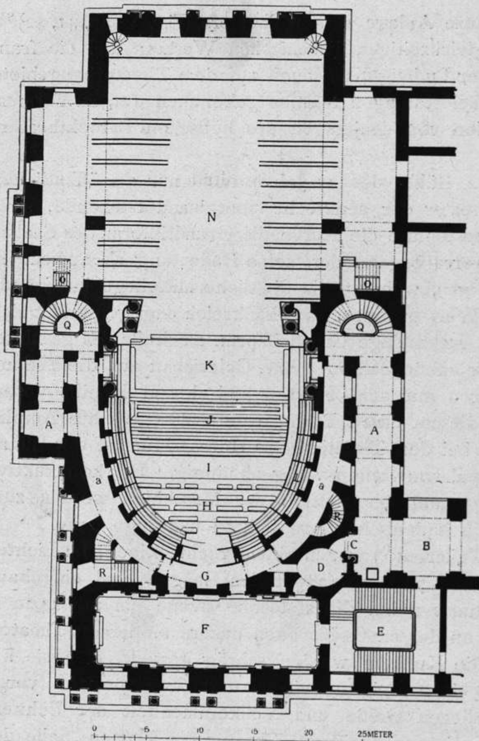
Fig. 43. Das Opernhaus im Schloß zu Versailles.
