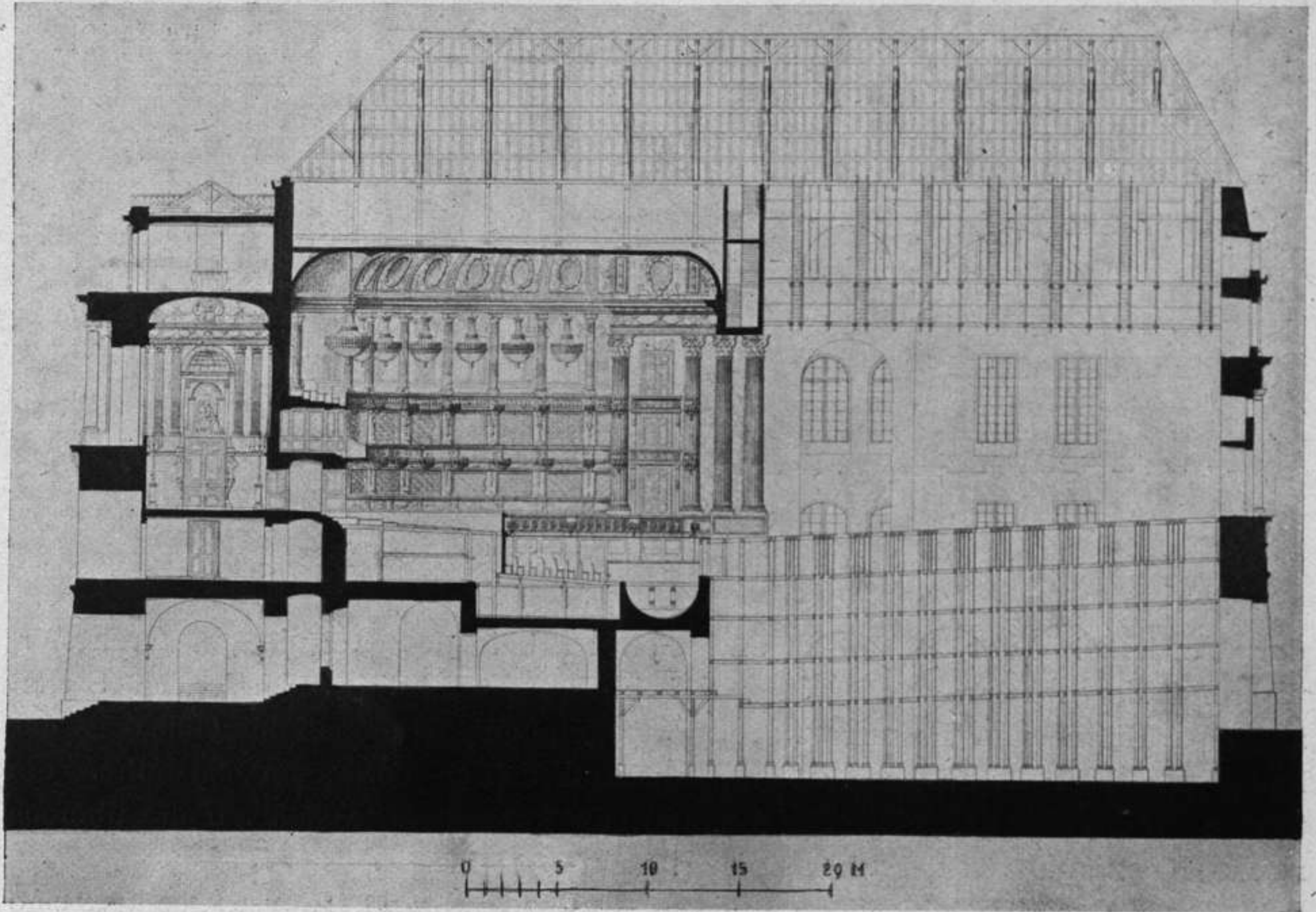
Fig. 46. Das Opernhaus zu Versailles: Längsschnitt.
