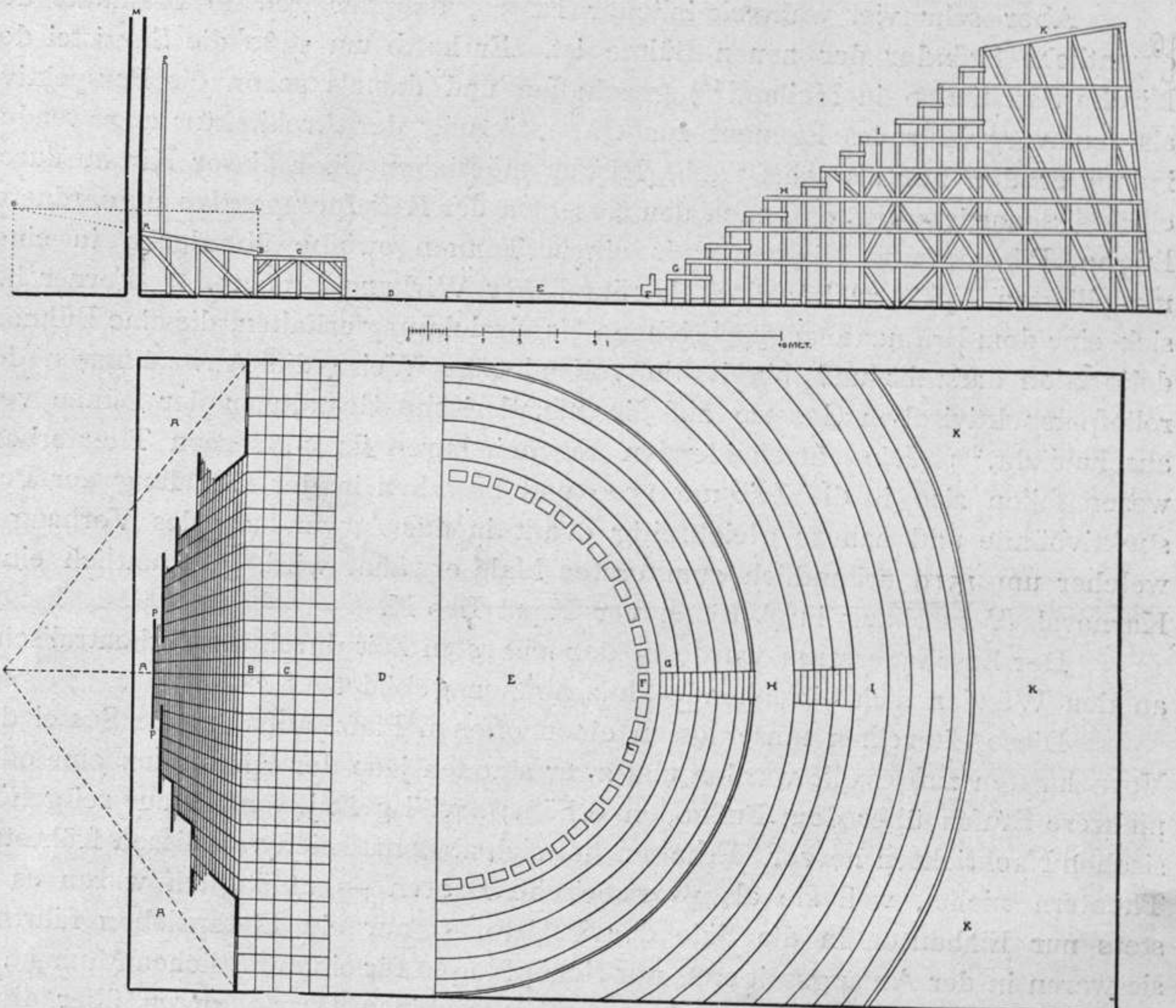
Fig. 4. Theateranlage in der ersten Hälfte des 16. Jahrhunderts. (Nach Originalplänen Serlios.)
