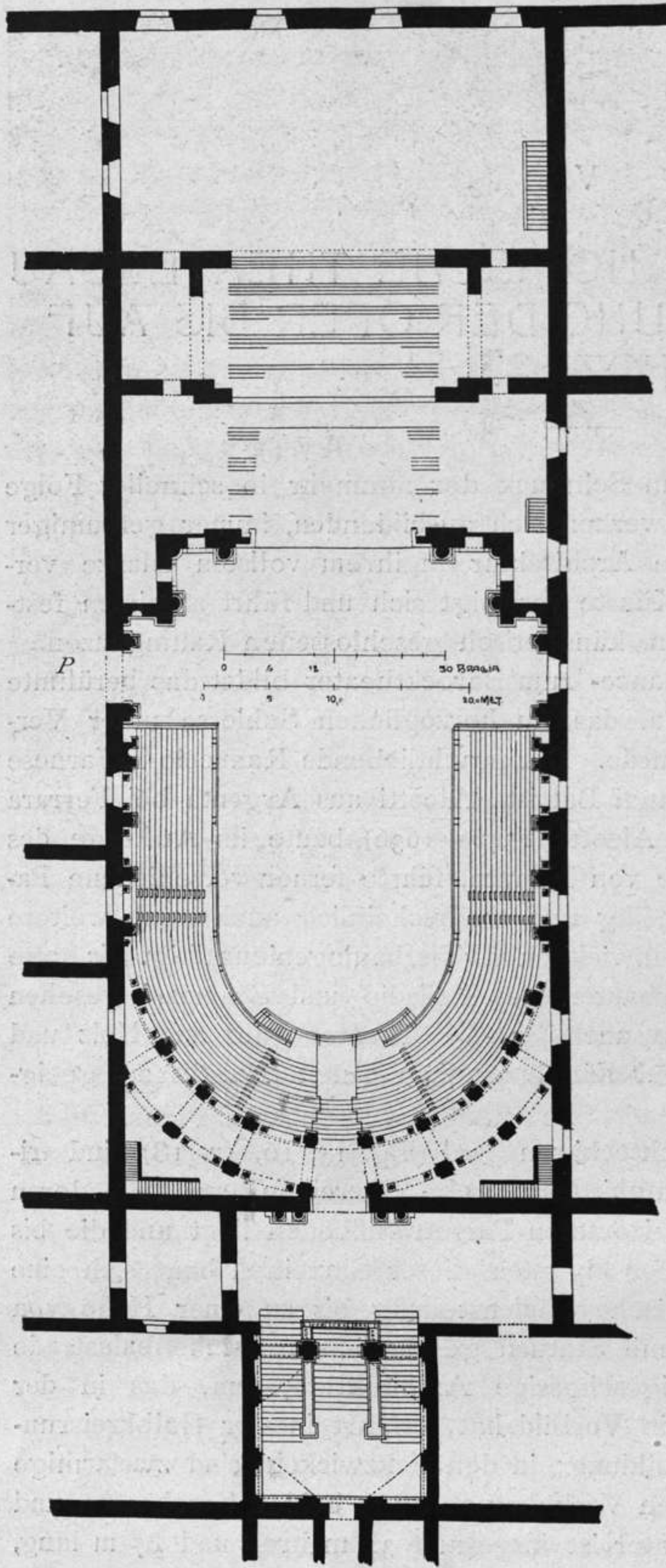
Fig. 15. Teatro Farnese in Parma. Grundriß.
