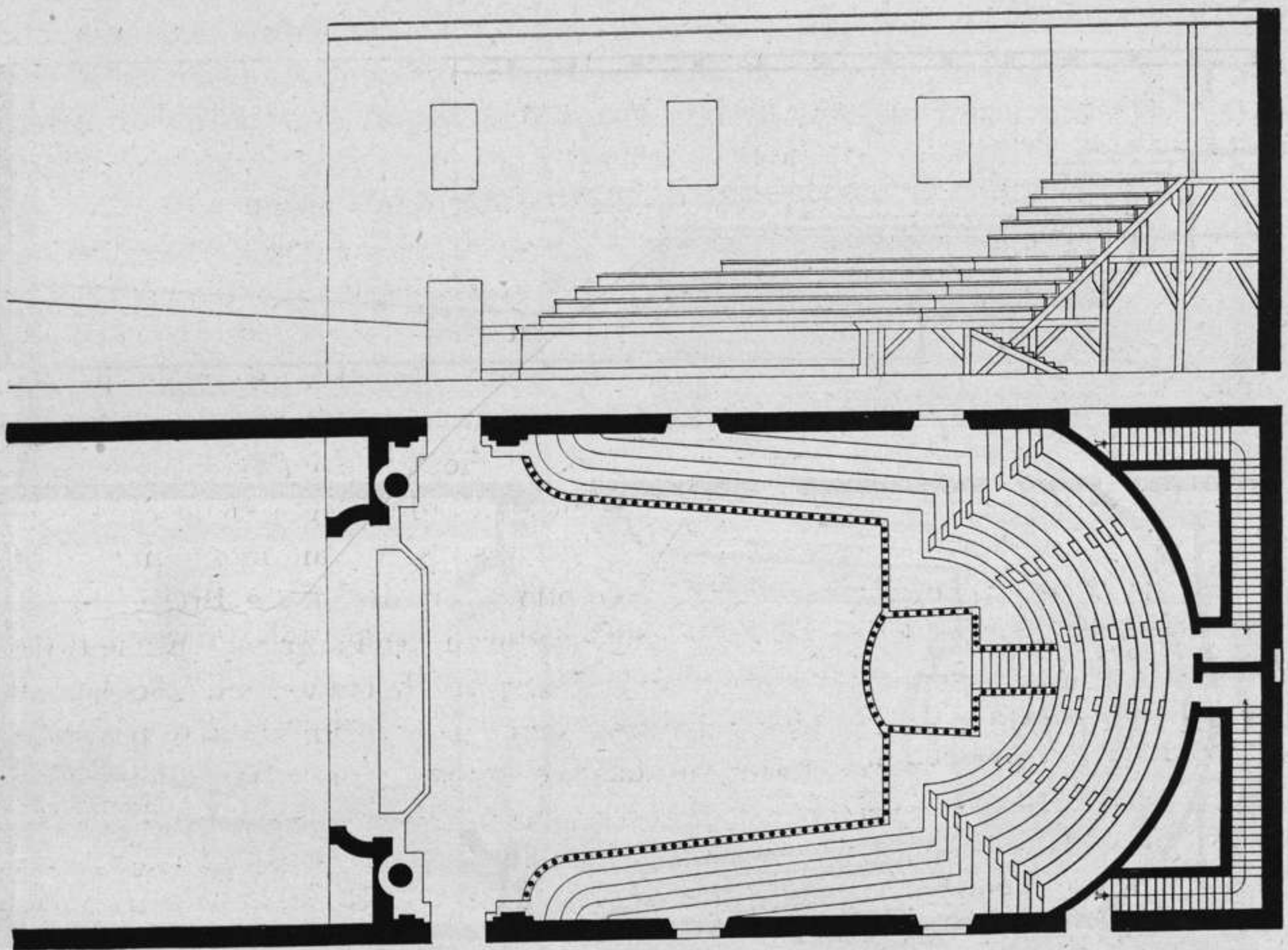
Fig. 19. Theatertypus nach Originalplänen des Fabricio Carini Motta.
