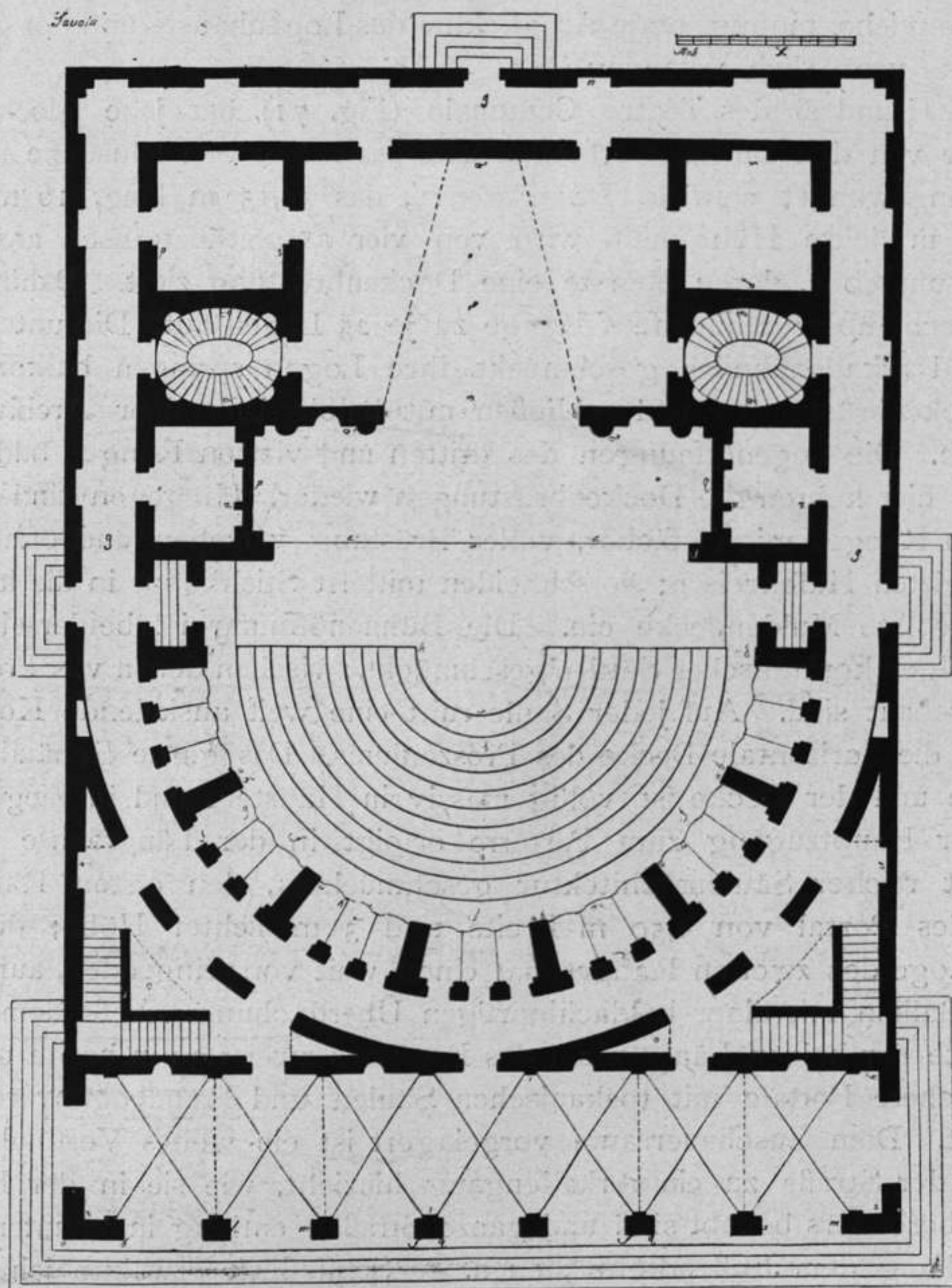
Fig. 72. Theaterprojekt von Vincenzo Arnaldi.
