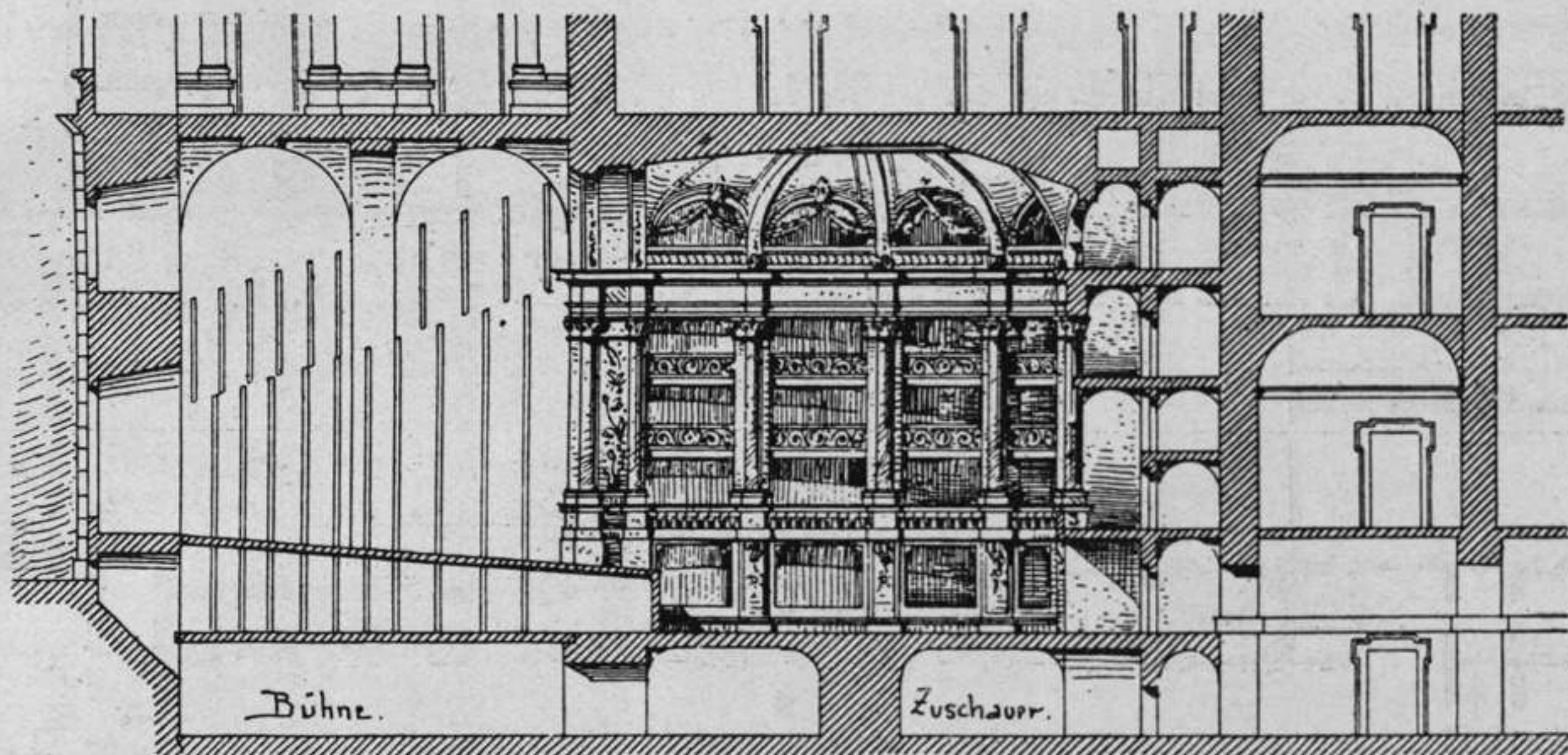
Fig. 66. Schloßtheater zu Caserta: Längenschnitt.
