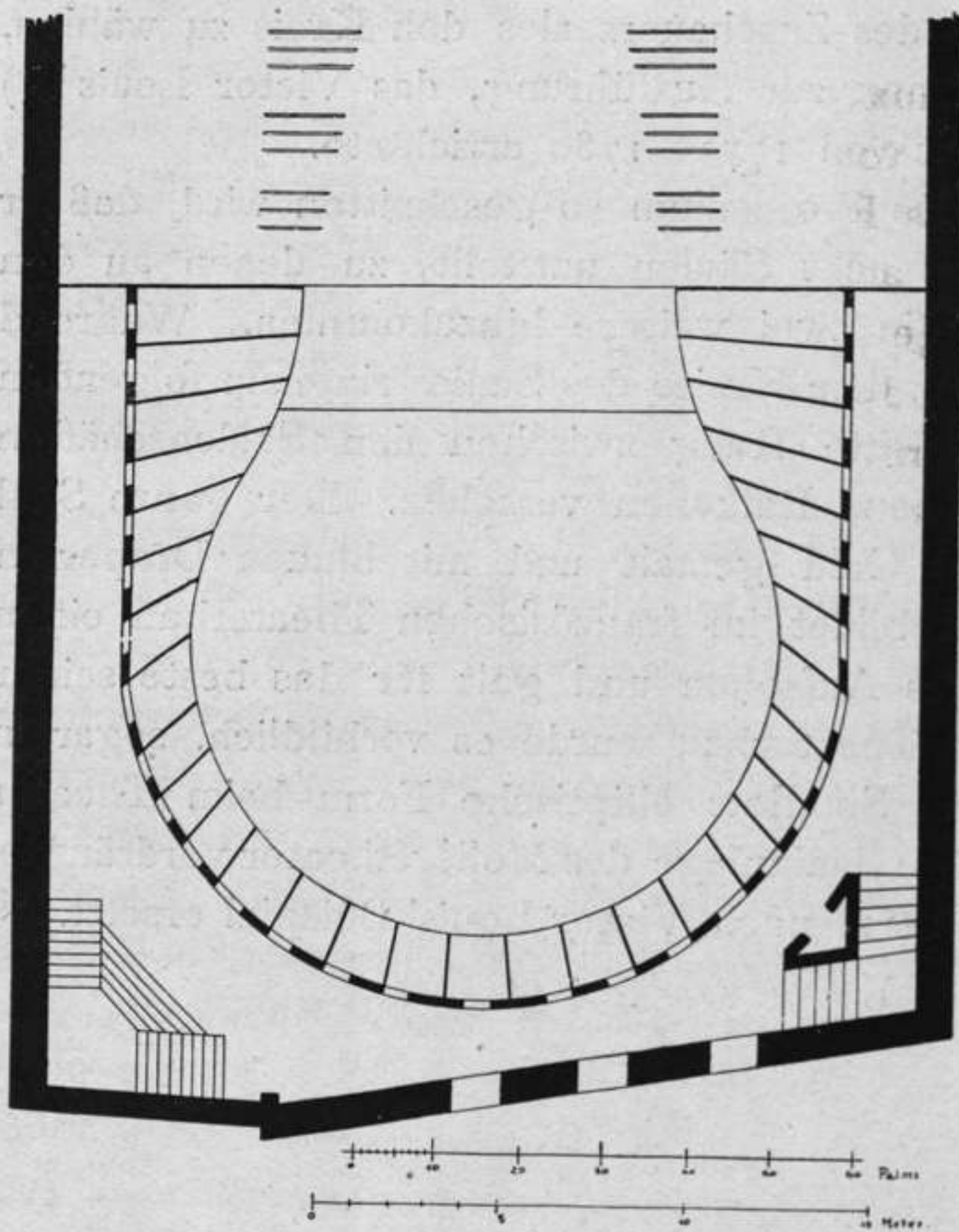
Fig. 50. Theater S. Benedetto in Venedig.
