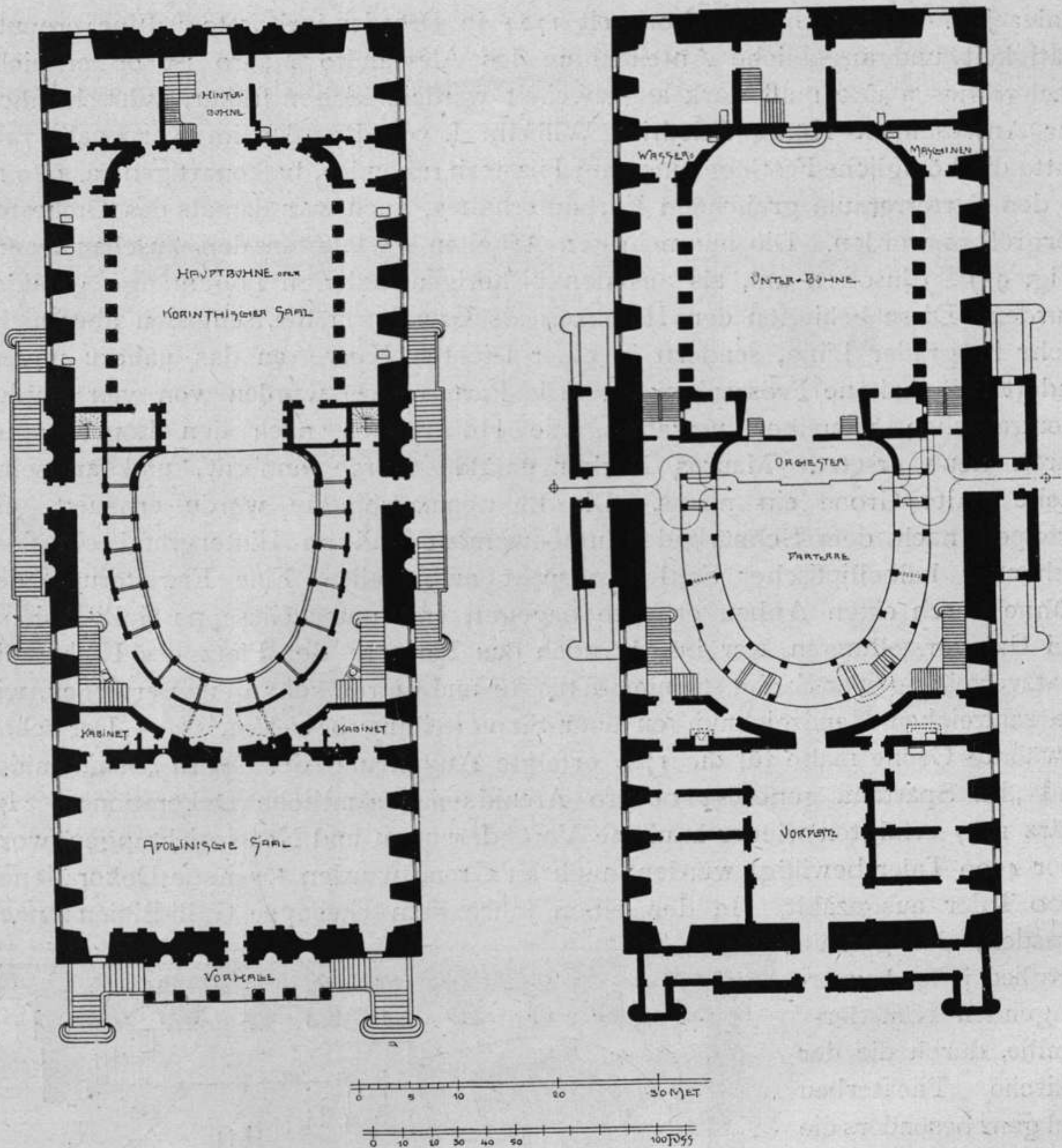
Fig. 94. Das alte Opernhaus in Berlin.
