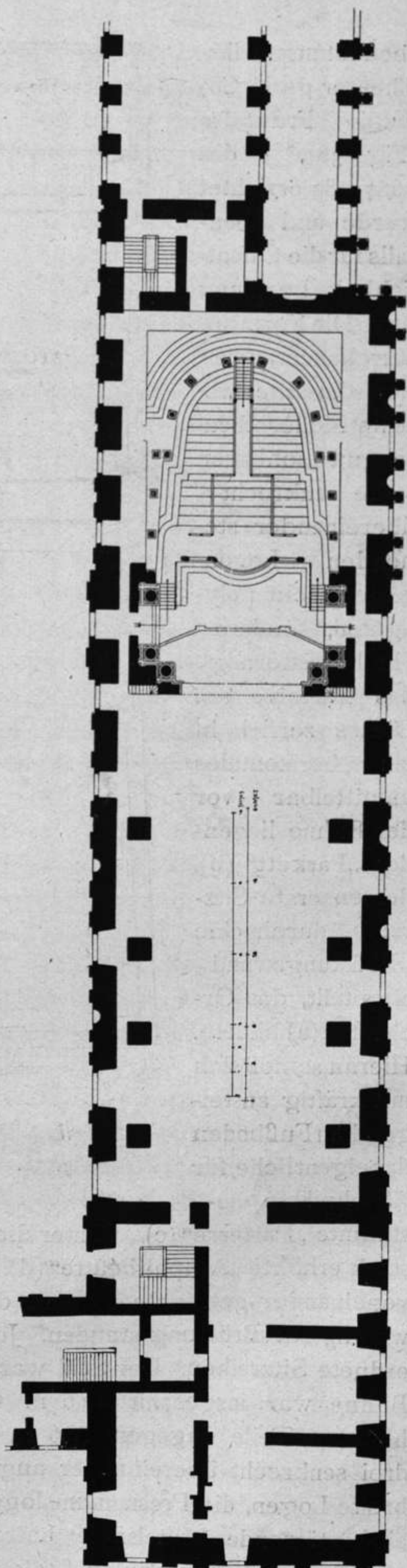
Fig. 39. Das Theater Ludwig XIV. in den Tuileries („Salle des machines“): Erdgeschoßgrundriß.
