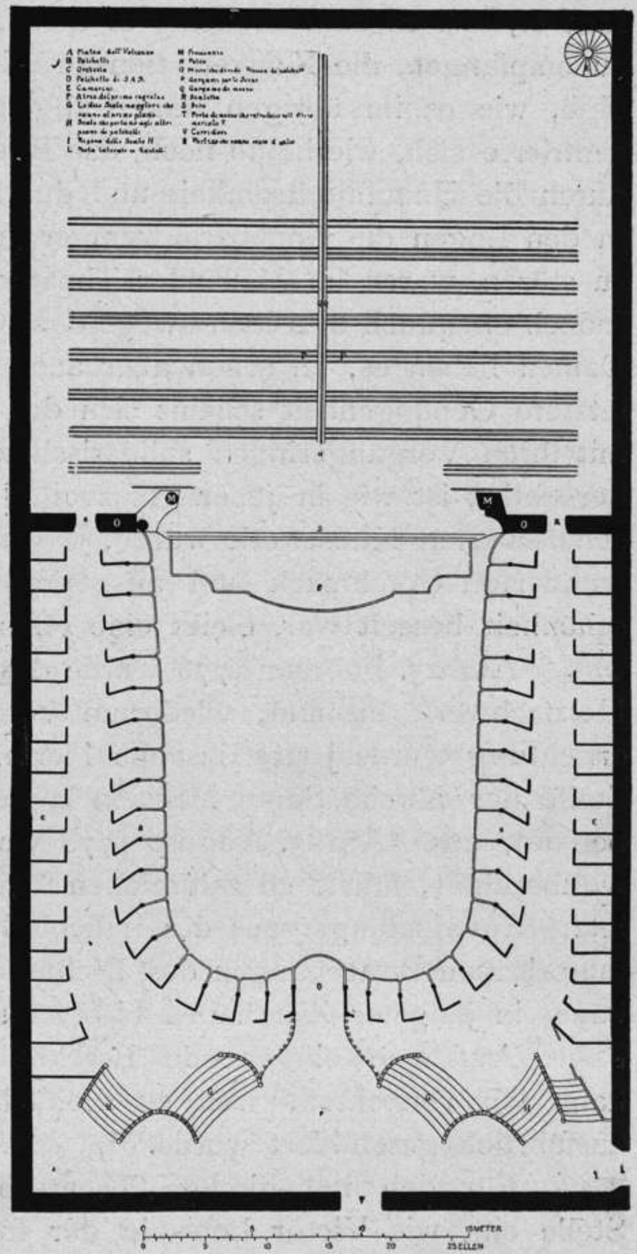
Fig. 75. Altes Theater in Mailand. [(Nach einer Handzeichnung.)]
